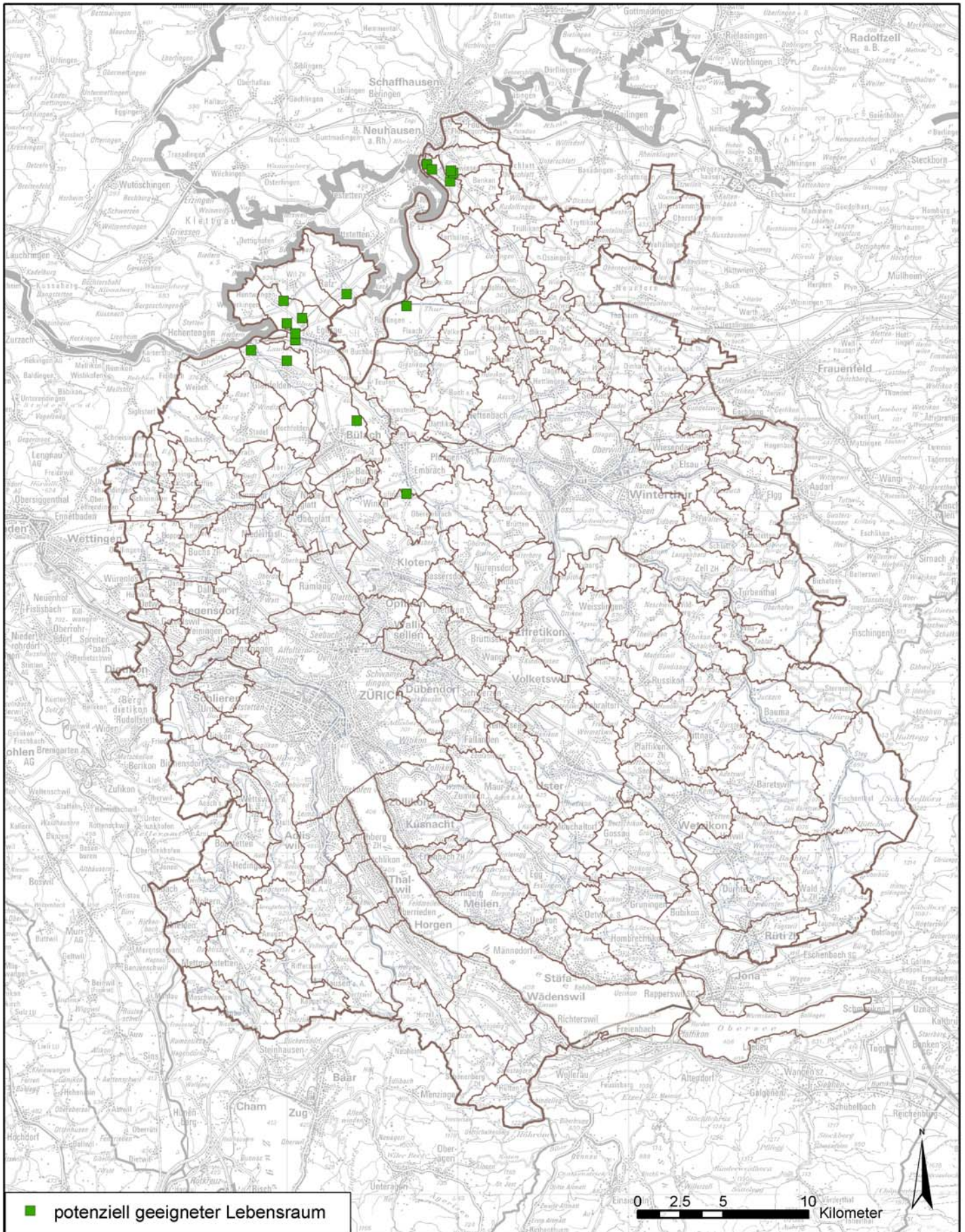
Karte der potenziell geeigneten neuen Lebensräume für Gagea pratensis im Kanton Zürich
