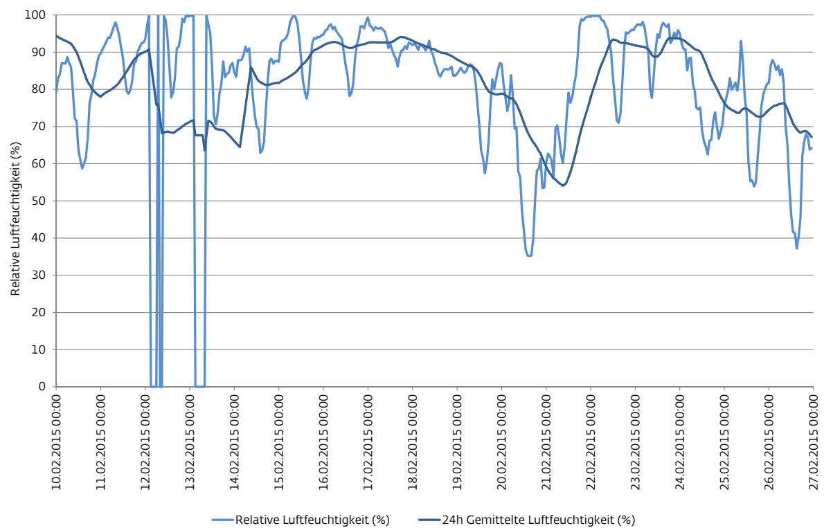
Abb. 46: Relative Luftfeuchtigkeit
