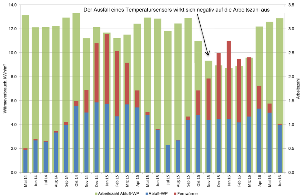
Abb. 14 : Kirchgasse 13: Spezifische Wärmeproduktion der Abluft-Wärmepumpe sowie Deckung der Spitzenlast über die Fernleitung (Fernwärme); Arbeitszahl der Abluft-Wärmepumpe; zwischen Oktober 2015 und März 2016 ist ein Temperatursensor in einem der zwei Verdampfer ausgefallen, was vorübergehend zu einer Reduktion der Arbeitszahl geführt hat
