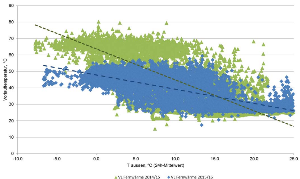
Abb. 15 Kirchgasse 13: Vorlauftemperatur Fernwärme vor und nach der Ausserbetriebssetzung des Heizölkessels
