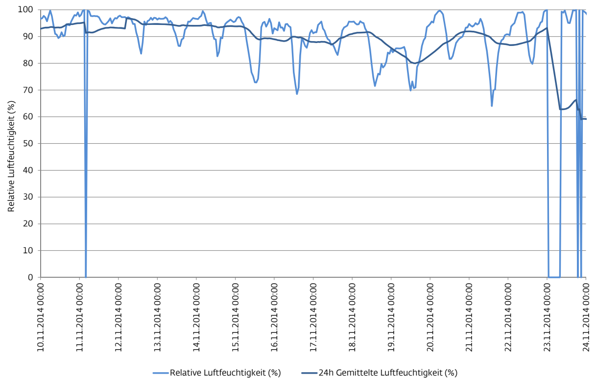
Abb. 44: Relative Luftfeuchtigkeit
