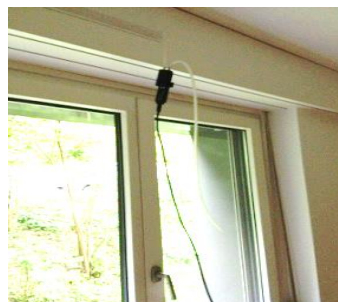
Abb. 27: Druckdifferenzmessung beim Aussenluftdurchlass
