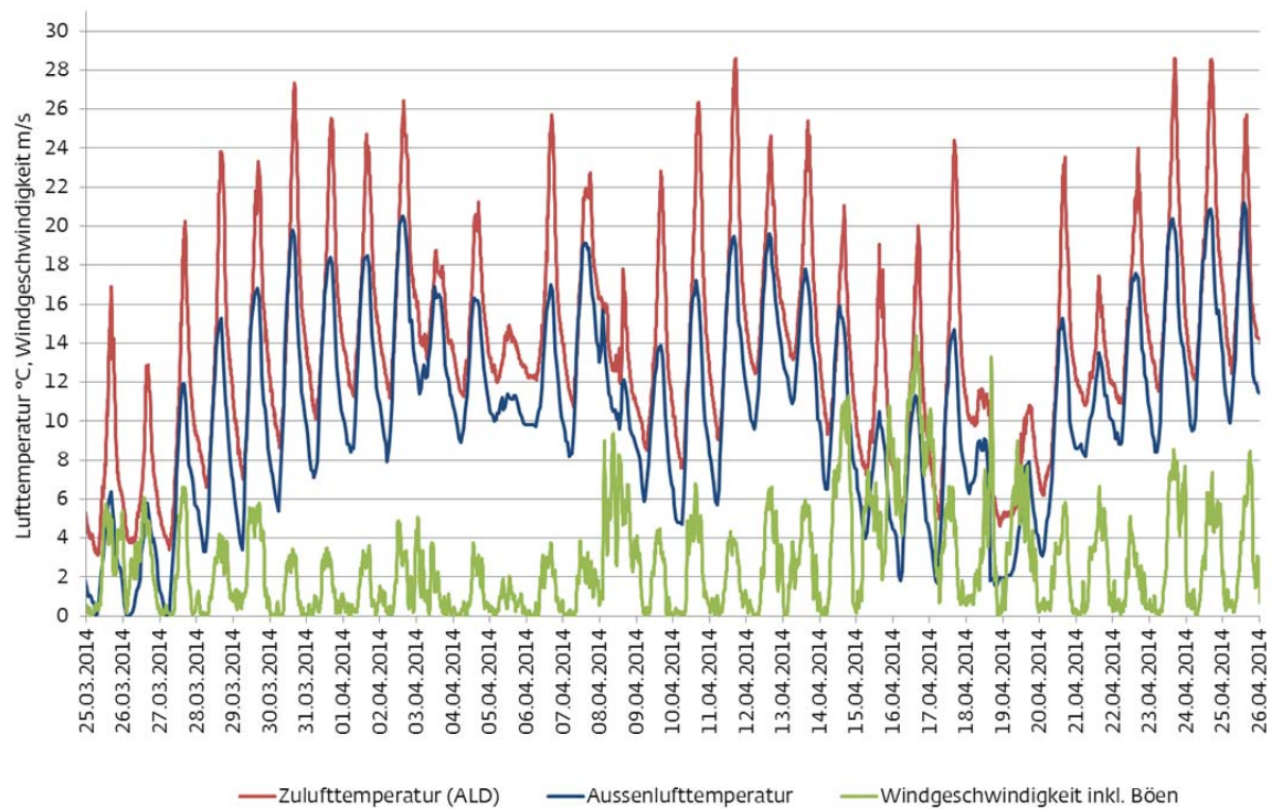
Abb. 21: Aussen- und Zulufttemperatur im Aussenluftdurchlass, raumseitig; Windgeschwindigkeit (Messung auf Dach). Eine Umkehrung der Strömungsrichtung von innen nach aussen tritt auch bei hohen Windgeschwindigkeiten und entsprechend stark variablen Druckverhältnissen auf der Fassade nie auf.
