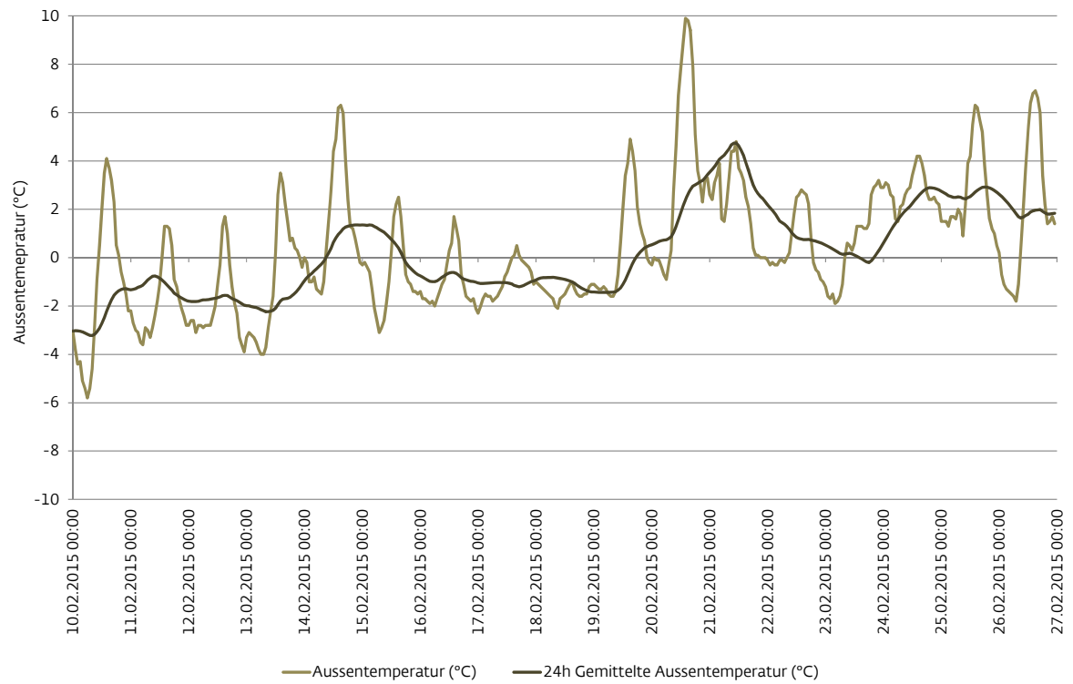
Abb. 45: Aussenlufttemperatur
