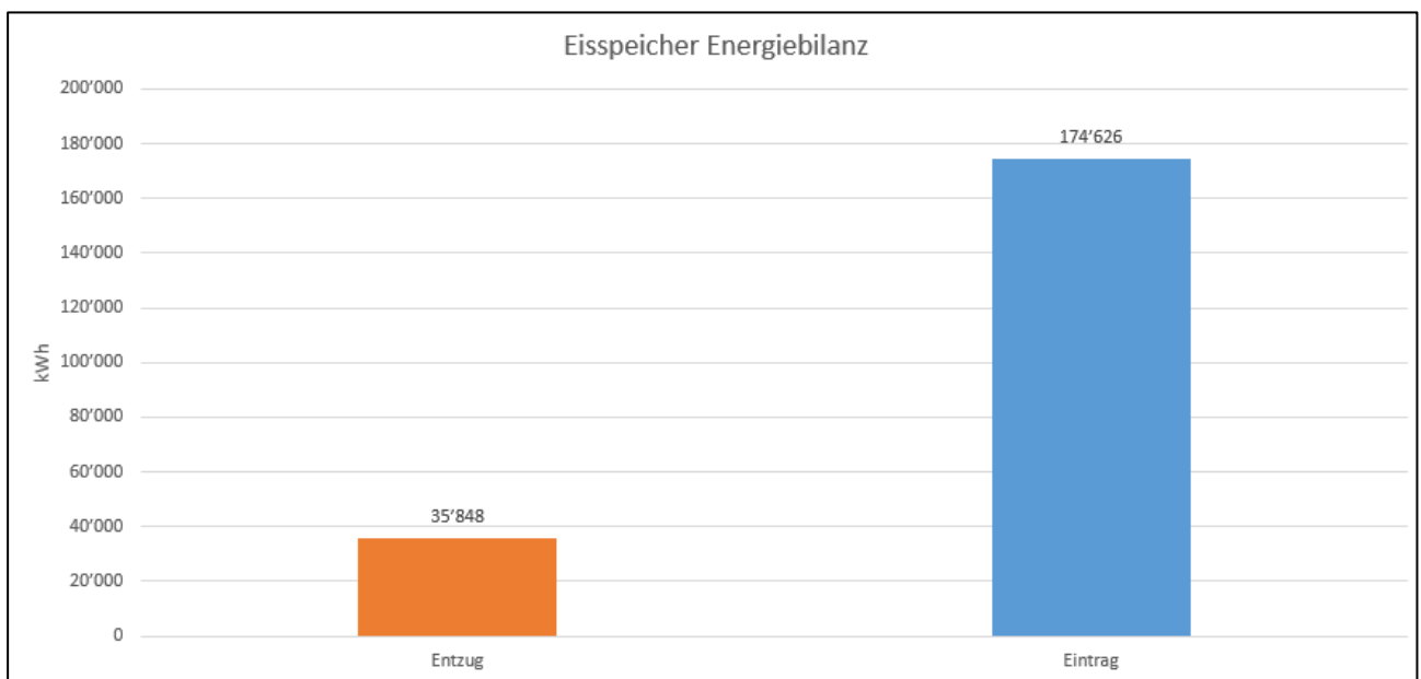
Abbildung 2-6: Bilanz Eisspeicher. Verhältnis zwischen Energieentzug und Energieeintrag.
