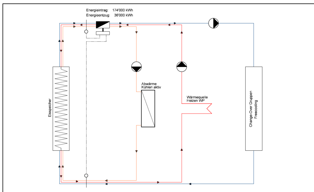
Abbildung 1-17: Durchfluss und Messprinzip des Eisspeichers.
