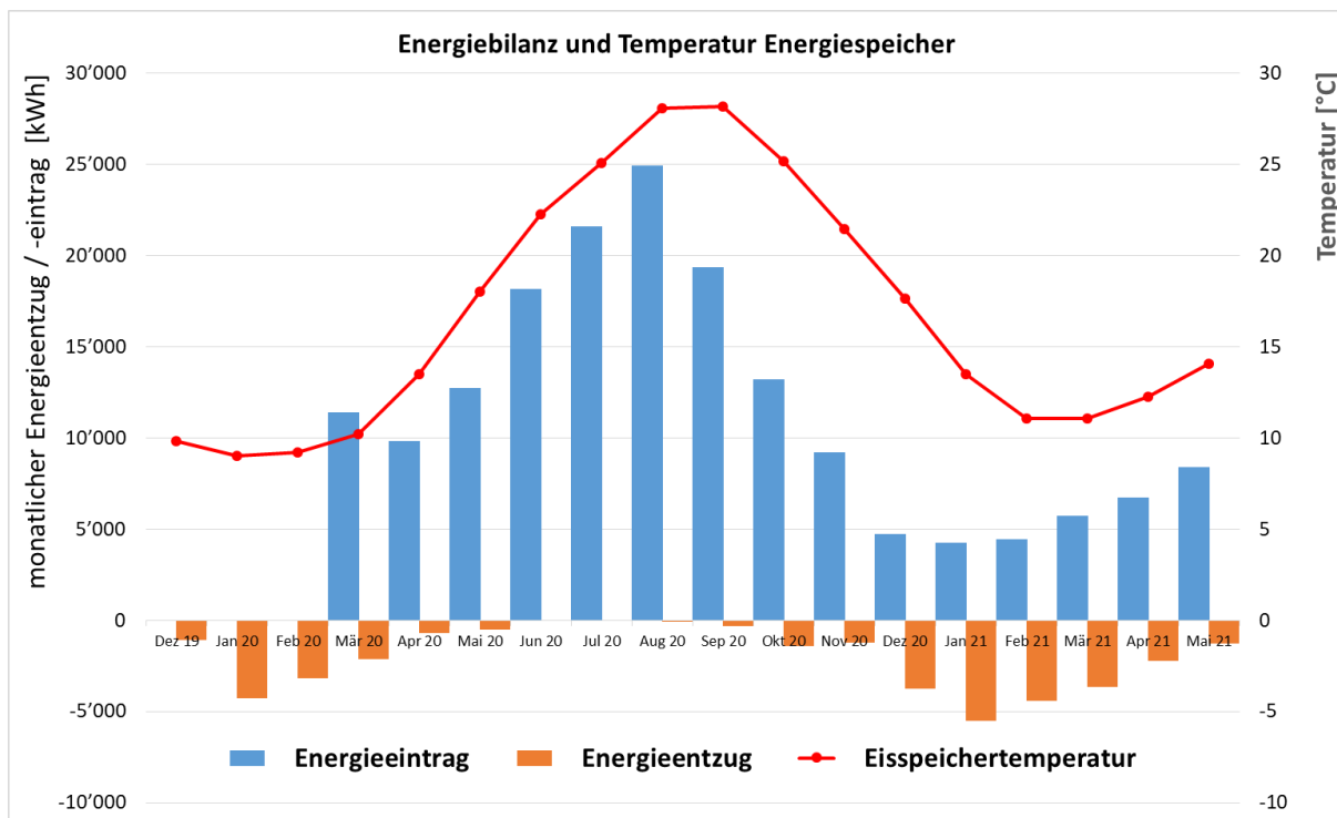
Abb. 2: Gemessene Energiebilanz und Temperaturen im Energiespeicher / Eisspeicher
