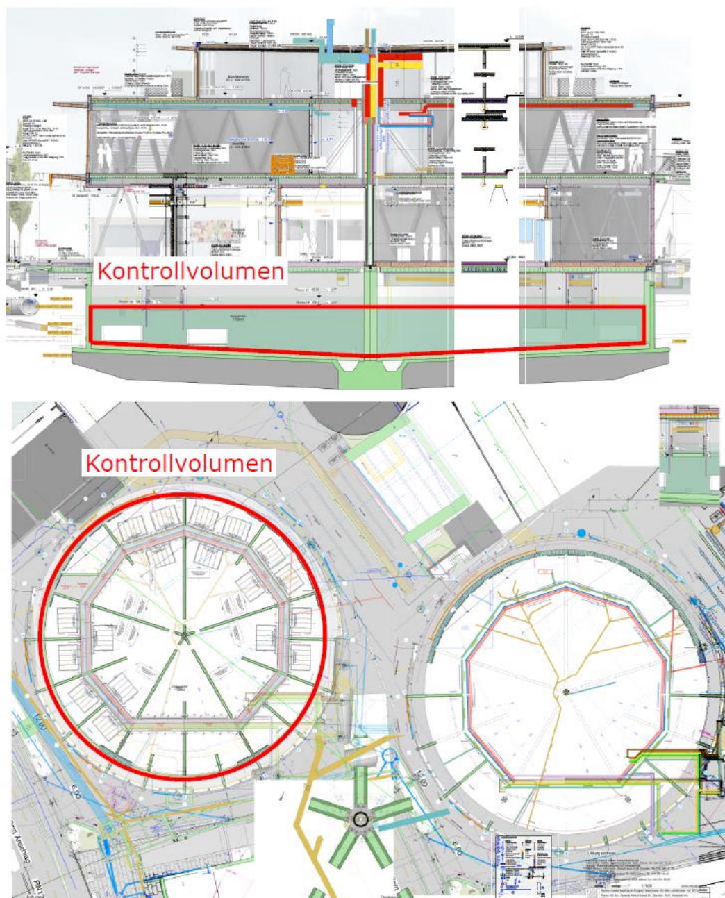
Abbildung 4-1: Kontrollvolumen des Eisspeichers für das thermische Eisspeichermmodell im Querschnitt und Grundriss
