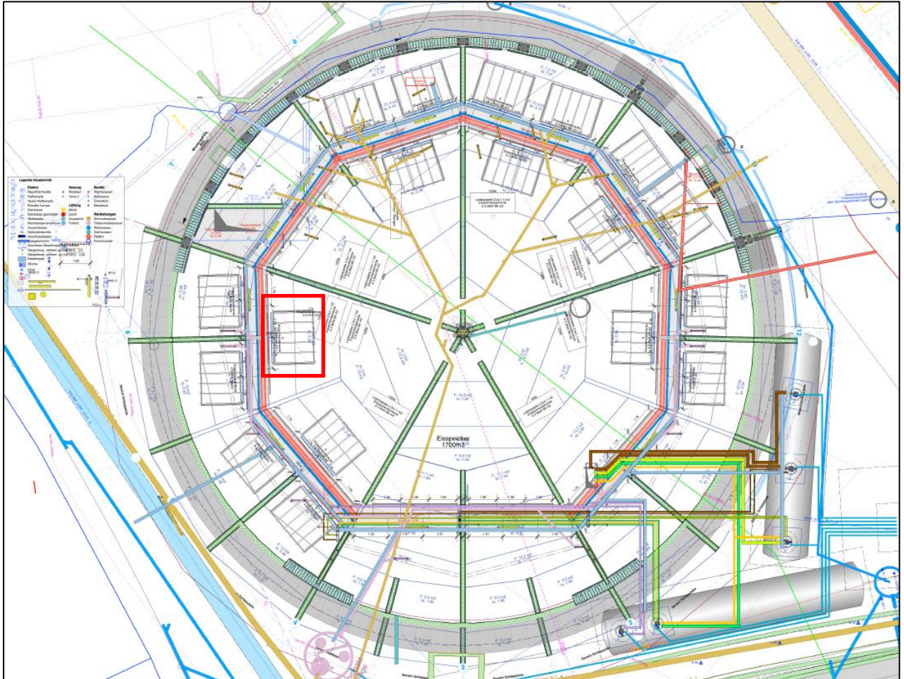
Abbildung 1-6: Sicht auf den Eisspeicher mit den verbauten Wärmetauschern (Paket rot markiert).
