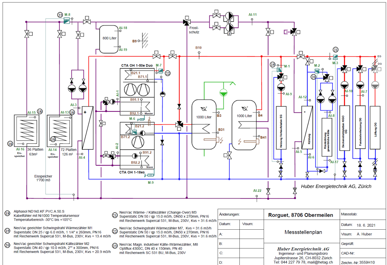
Abbildung 1-15: MSR-Schema und Messstellenplan
