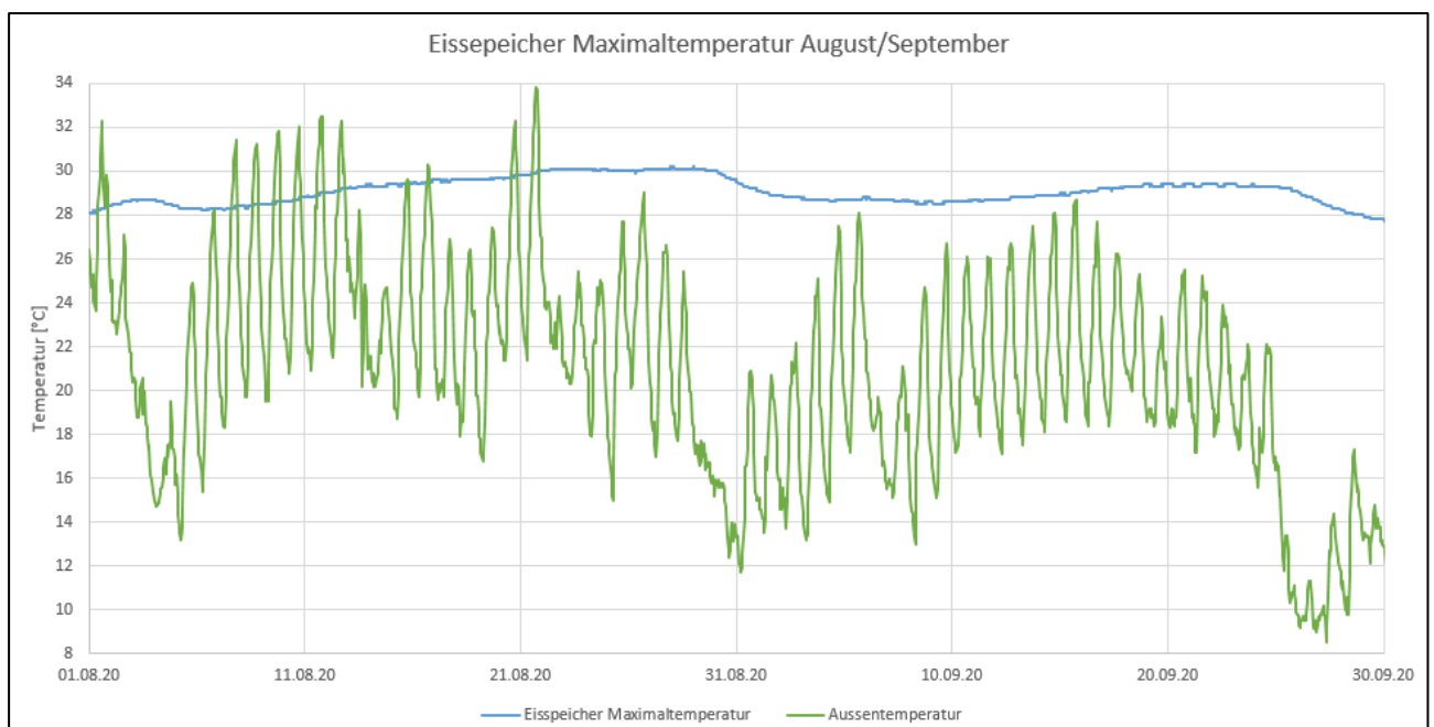
Abbildung 2-9: Temperaturverlauf im Eisspeicher und Aussentemperatur August/September 2020
