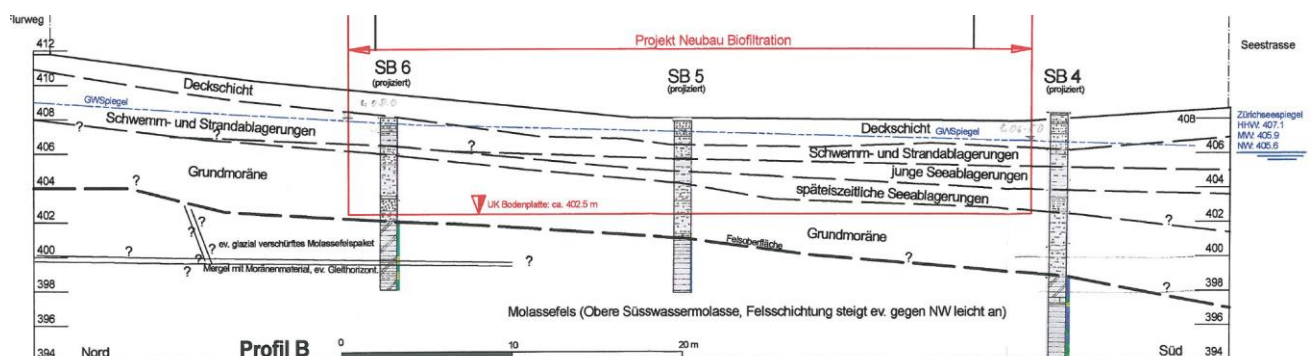
Abbildung 2-2: Auszug aus der Baugrunduntersuchung der ARA Meilen (Dr. Vollenweider AG, Juni 2008)
