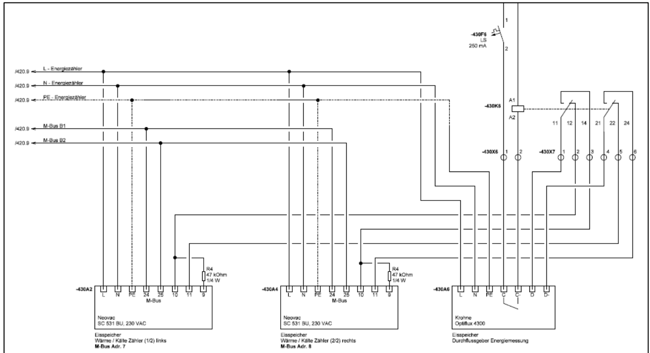
Abbildung 1-16: Ausschnitt aus dem MSR-Anschlussschema. Anschluss der beiden Rechenwerke und des Durchflussgebers zur Energiemessung des Eisspeichers
