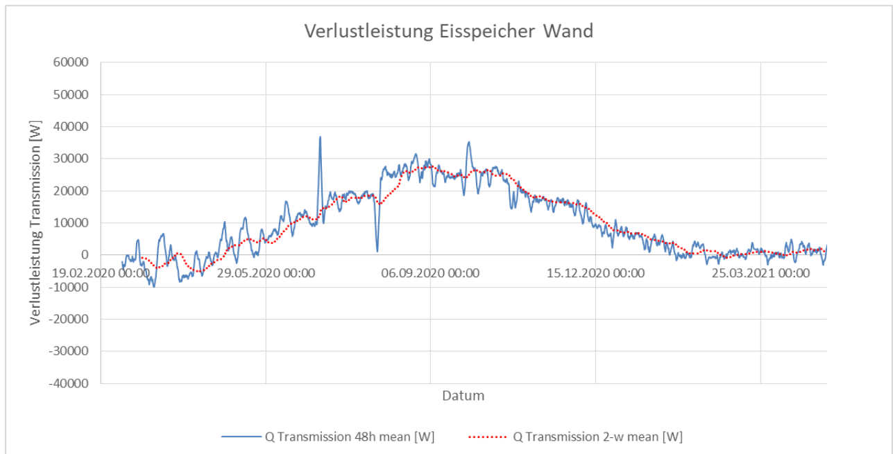
Abb. 3: Wärmeaustausch des Energiespeichers mit dem Umgebenden Erdreich ermittelt mittels Modell aus den Messwerten.
