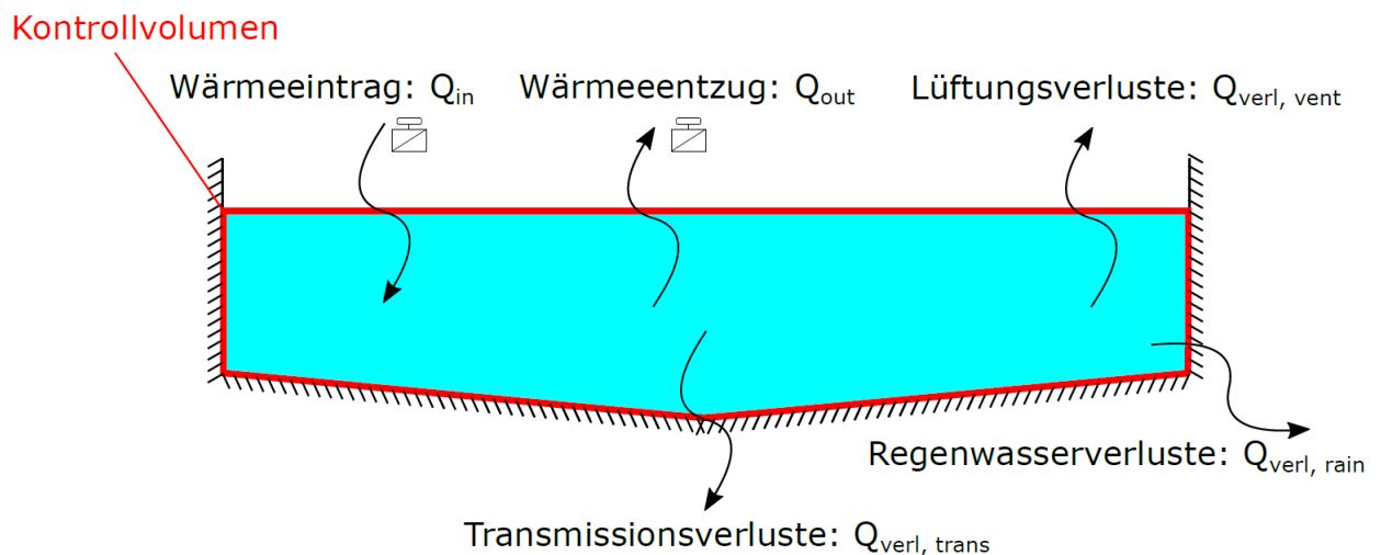
Abbildung 4-2: Kontrollvolumen des Eisspeichers mit Wärmeströme und Richtung der Wärmeströme gemäss Konvention im Modell
