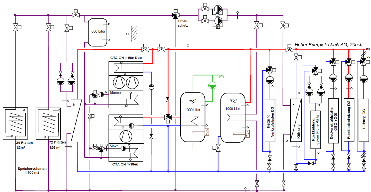
Abb. 1: Schema der Wärme- und Kälteerzeugung und der hydraulischen Einbindung des Energiespeichers.
