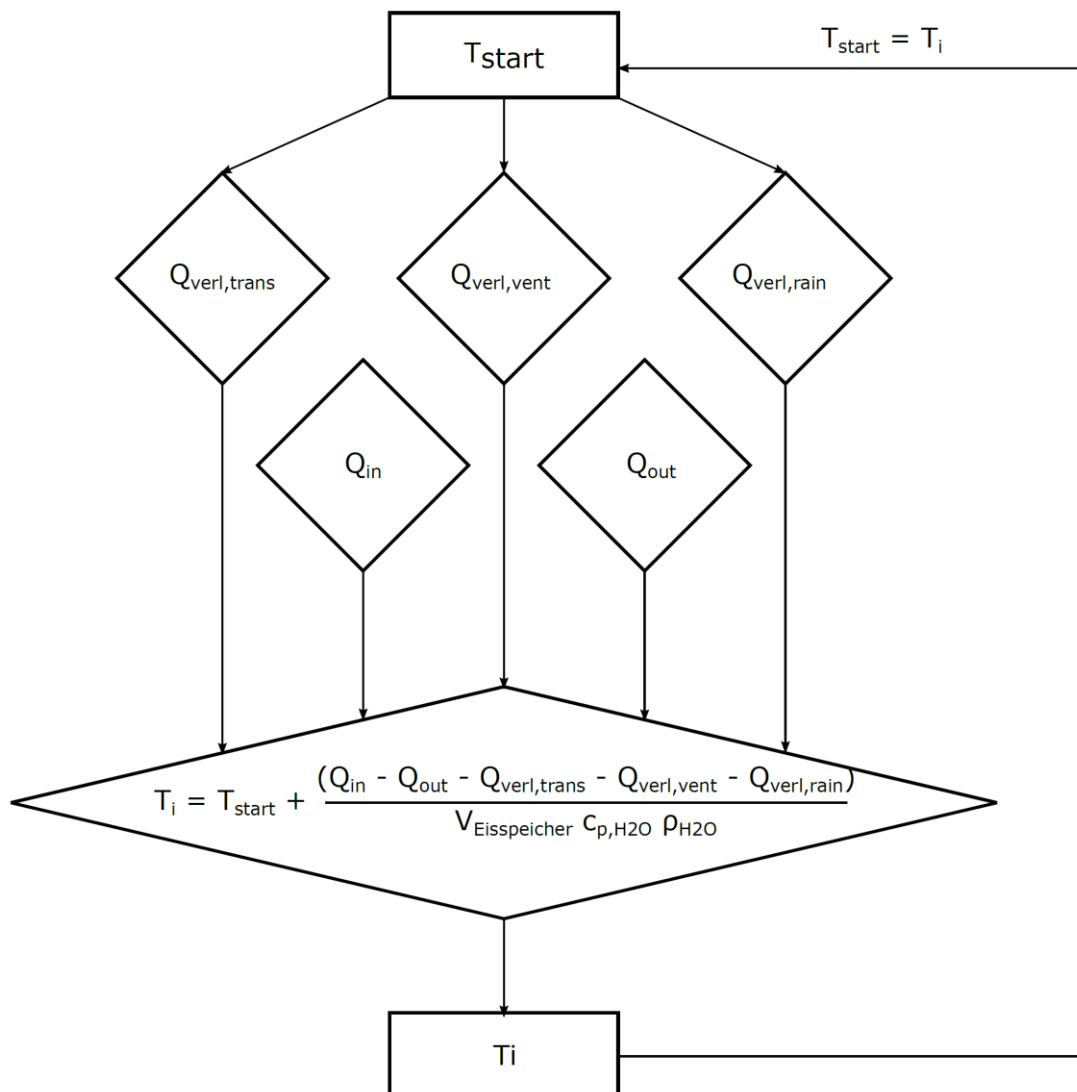
Abbildung 4-3: Beschreibung der Berechnung der Temperatur zum Zeitpunkt i im thermischen Modell des Eisspeichers.
