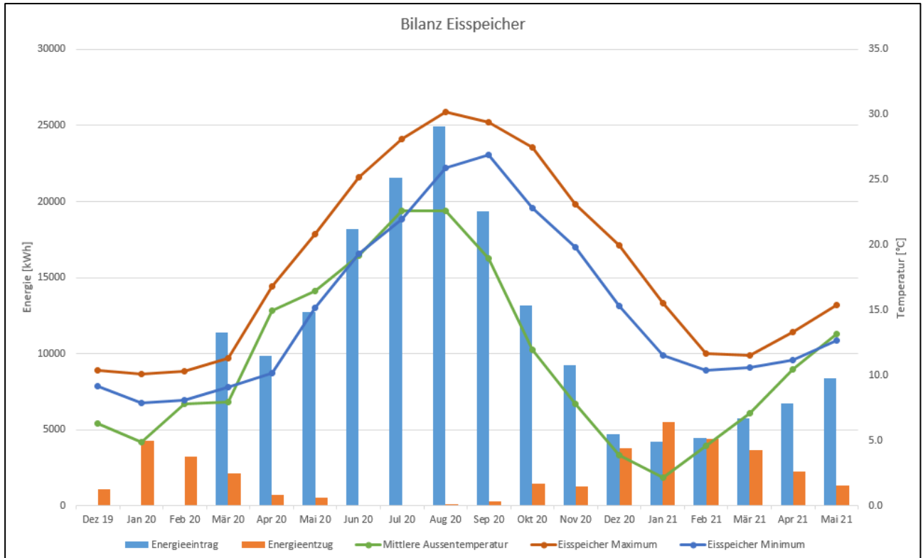
Abbildung 2-5: Bilanz Eisspeicher. Min/Max Temperaturen, Energieeintrag- und Entzug sowie mittlere Aussentemperatur.
