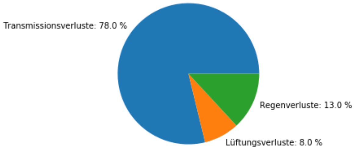
Abb. 4: Wärmeverluste des Energiespeichers Rorguet in der Jahresbilanz
