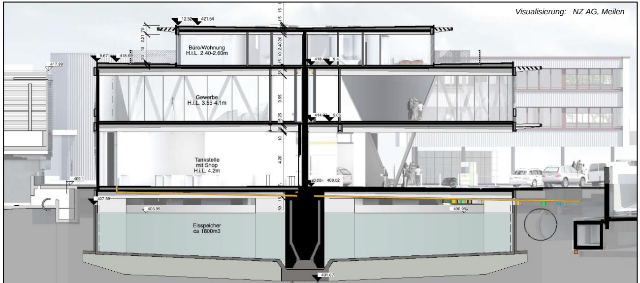
Abbildung 1-4: Ausschnitt aus der Konzeptphase. Schnitt durch das Gebäude. Das ehemalige Klärbecken im Untergeschoss wird als Eisspeicher genutzt.
