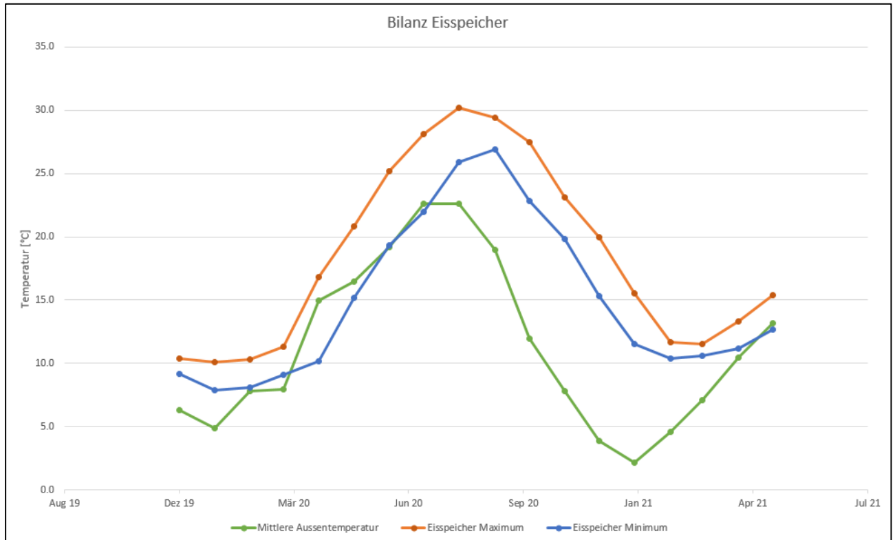
Abbildung 2-8: Temperaturverlauf im Eisspeicher und Aussentemperatur August 2019 bis Juli 2020
