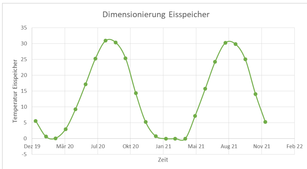
Abbildung 2-4: Berechneter Temperaturverlauf der mittleren Eisspeichertemperaturen mit einer Worst-Case Energiebilanz für den Heizbetrieb (fehlende Abwärme aus Gewerbekälte).
