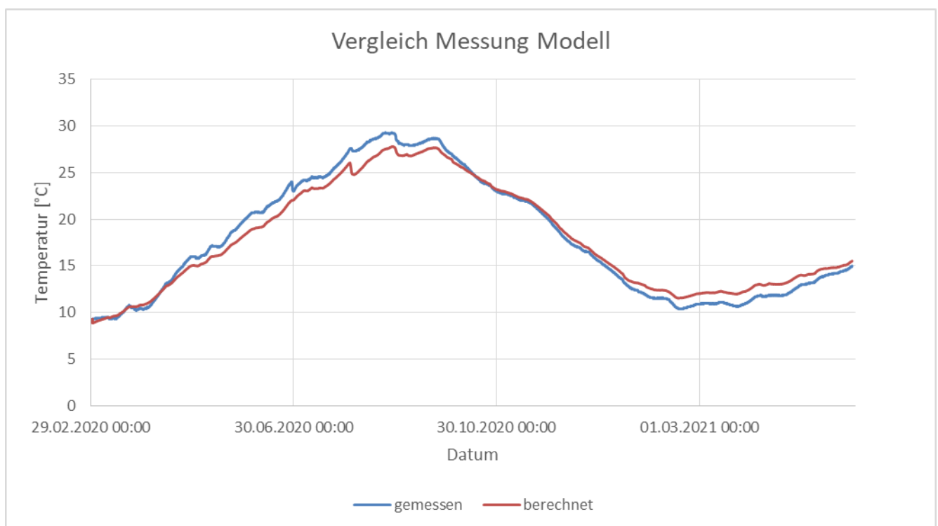
Abbildung 4-4: Vergleich gemessenen Eisspeichertemperatur und der modellierten Temperatur im Eisspeicher mit Vorgabe der gemessenen Eintrags- und Entzugsenergien.
