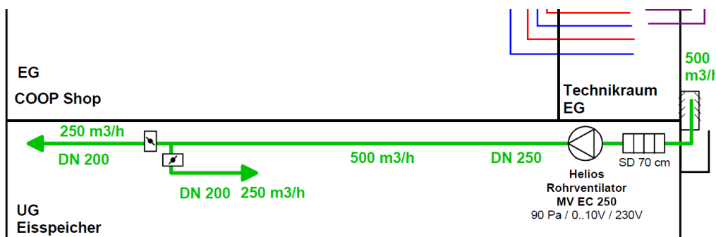
Abbildung 1-7: Lüftungsschema Zuluft Eisspeicher: Verhinderung von Gerüchen und Gewährleistung Frischluft.
