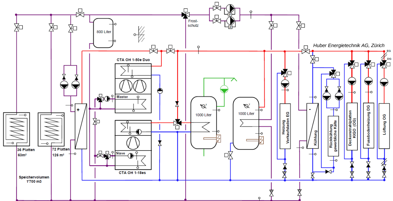
Abbildung 1-14: Hydraulisches Schema der Wärme- und Kälteerzeugung mit Energiespeicher / Eisspeicher
