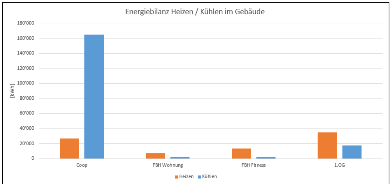
Abbildung 2-7: Bilanz Energiebedarf des Gebäudes.
