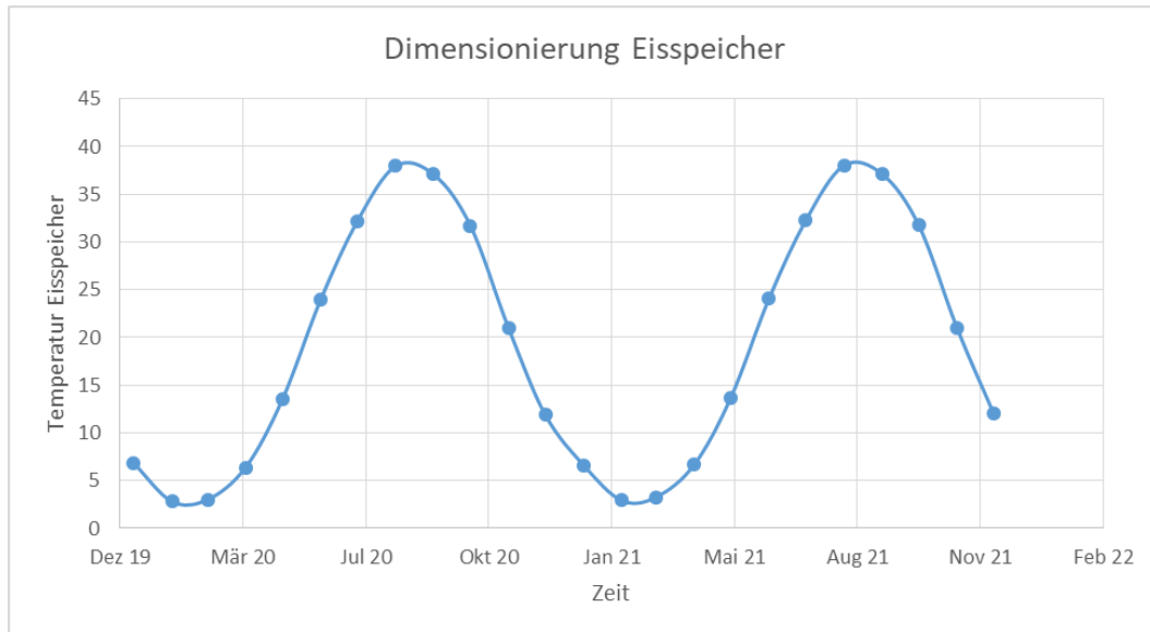
Abbildung 2-3: Berechneter Temperaturverlauf der mittleren Eisspeichertemperaturen mit Energiebilanz aus der Projektphase mit Kältebedarf gemäss Angabe Lebensmittelladen
