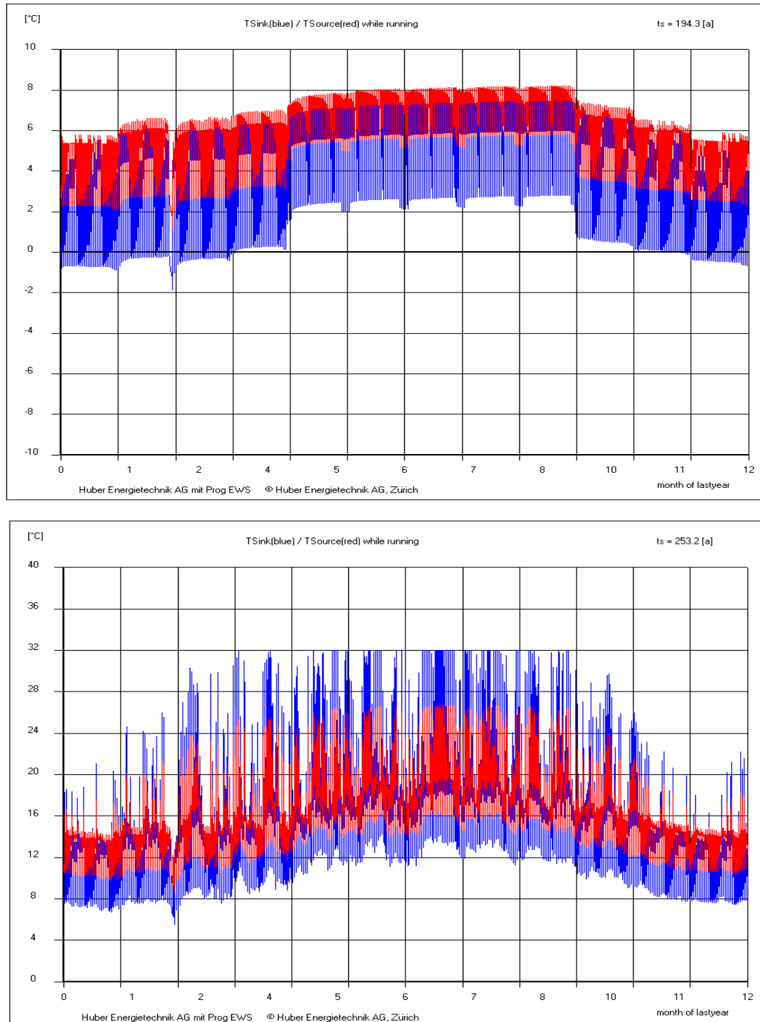
Abbildung 4.2: Jährlicher Temperaturverlauf im 50. Betriebsjahr für die Sondereintrittstemperatur (blau) und -Austrittstemperatur (Quellentemperatur, rot). Die Werte für das Haus A1 (oben) liegen über das ganze Betriebsjahr weit unter den Werten für das Haus B2 (unten). Die Skalen auf der Ordinate sind unterschiedlich.
