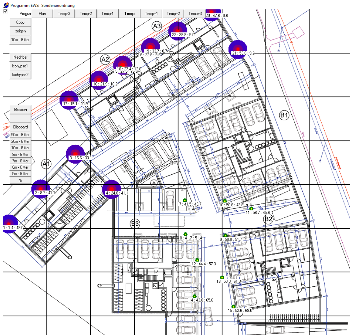
Abbildung 8.5: Sondenanordnung A-Häuser.
