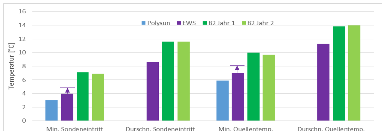
Abbildung 5.3: Vergleich Eintritt- und Austritttemperaturen Erdwärmesonde. Die EWS und Polysun Werte beachten beide einen Auslegungsfall, welcher in den 2 Jahren aber nicht stattfand. Die Minimaltemperaturen des EWS ohne Auslegungsfall werden von den zwei Pfeilen markiert.
