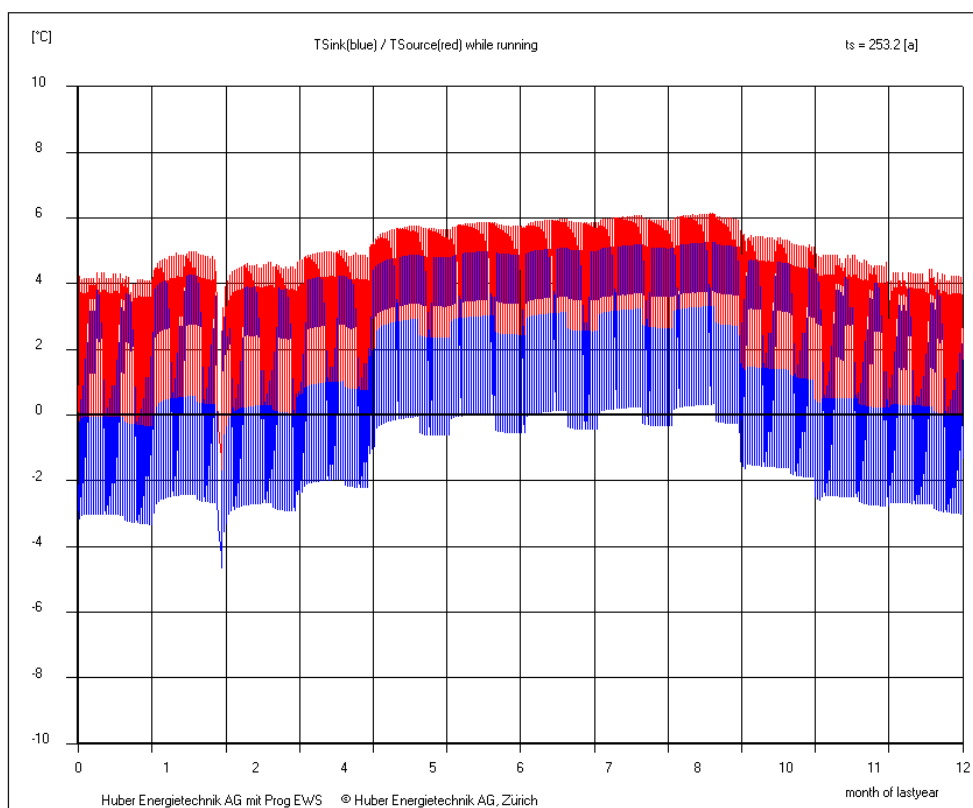
Abbildung 8.7: Jährlicher Temperaturverlauf für Sondereintritt (blau) und Quelltemperatur (rot) im 50. Betriebsjahr für das Haus B2 mit Regeneration (oben) und ohne Regeneration (unten). (unterschiedliche-Skala beachten)
