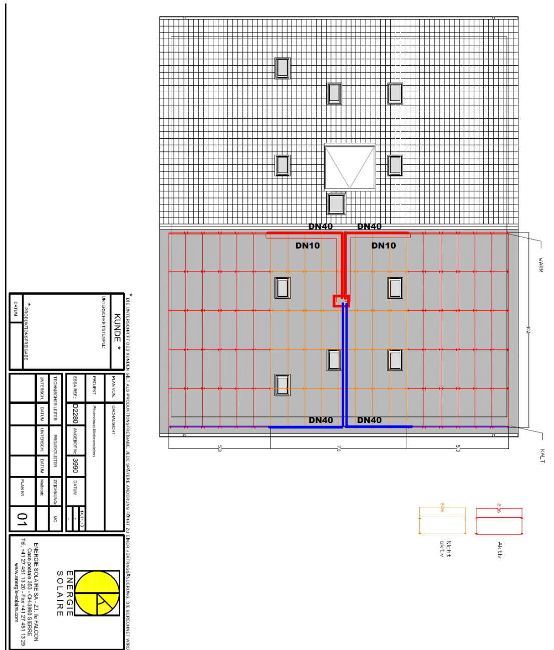
Abbildung 2.1: Unverglaste Kollektoren von Energie Solaire SA auf den Häusern B1, B2 und B3 mit je 110 m 2 Absorberfläche
