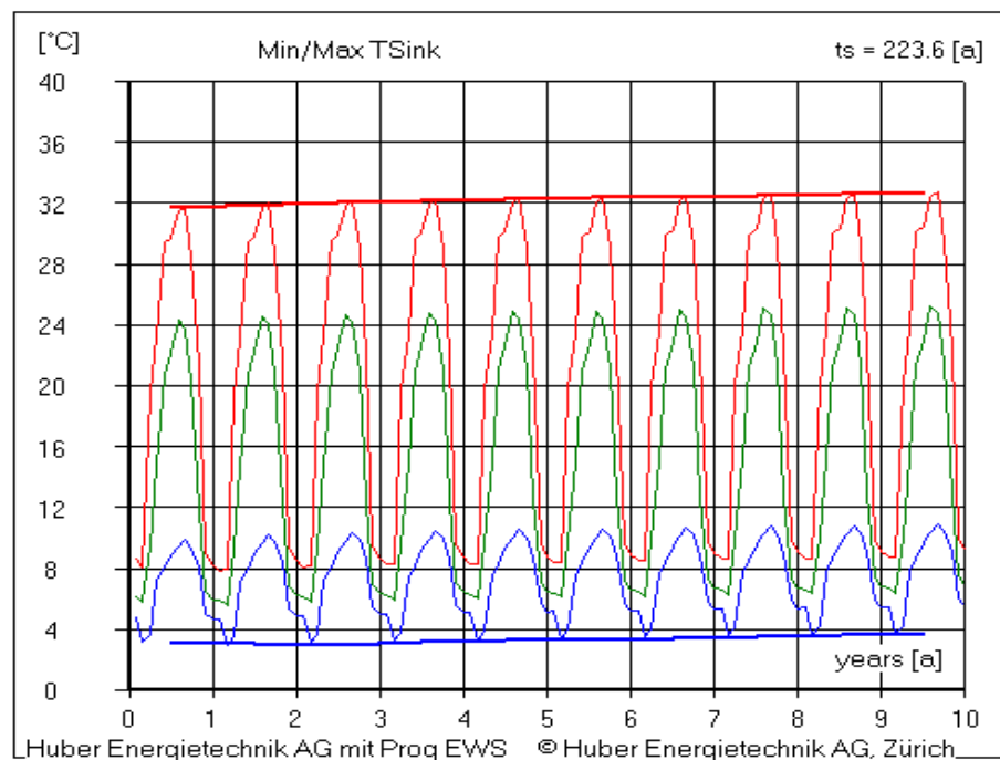
Abbildung 2.6: Sondereintritts- und Sondaaustrittstemperaturen. Simulation über 10 Jahre
