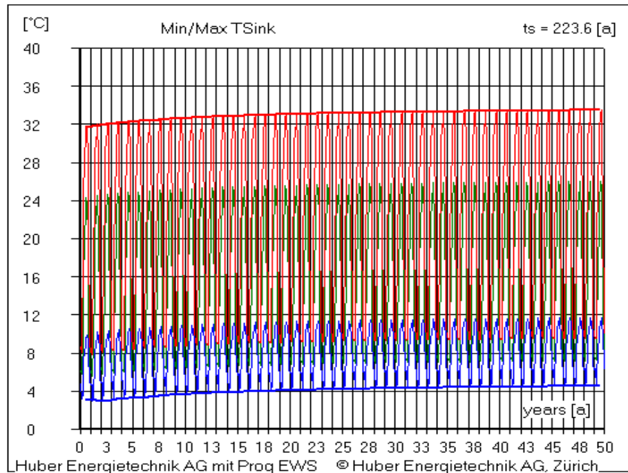
Abbildung 2.5: Sondereintritts- und Sondaaustrittstemperaturen Simulation über 50 Jahre (Diese Grafik stellt den Verlauf vor der Optimierung dar, mit maximaler Sondereintrittstemperatur auf 35 °C beschränkt)
