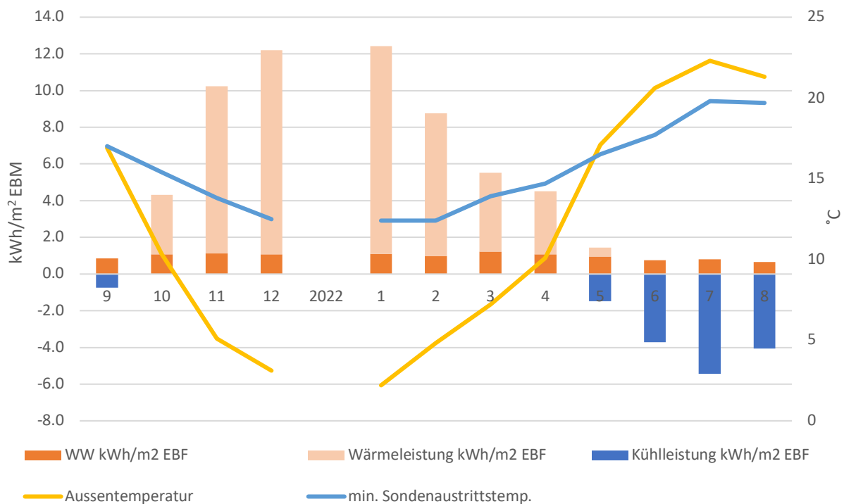
Abbildung 2: Monatliche Heizleistung für Heizwärme, Warmwasser und Kühlleistung sowie Aussentemperatur und die minimale Sondaaustrittstemp. Kühlleistung Haus negativ dargestellt.
