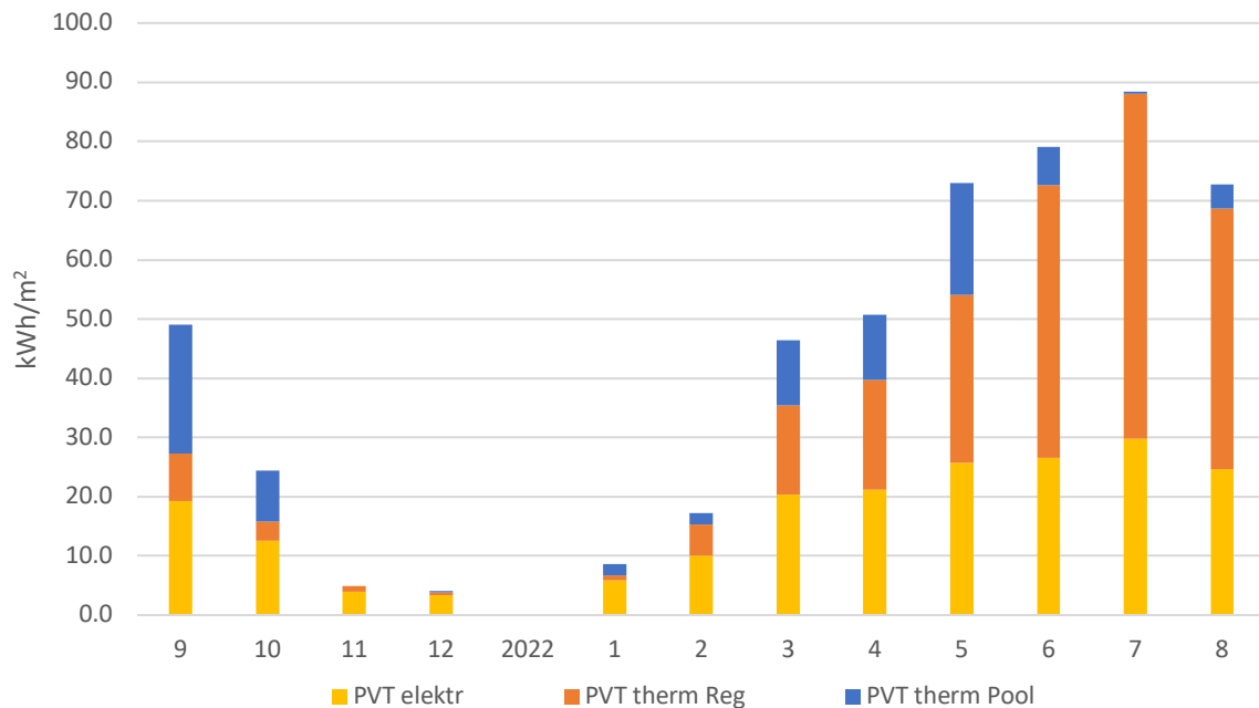
Abbildung 6: Ertrag Hybridkollektor pro m 2 Kollektorfläche: elektrischer Ertrag (gelb), thermischer Ertrag zur Sonde (orange) und thermischer Ertrag zum Schwimmbad (blau)
