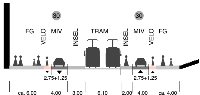
Strassenprofile Rämistrasse, Mittellage
