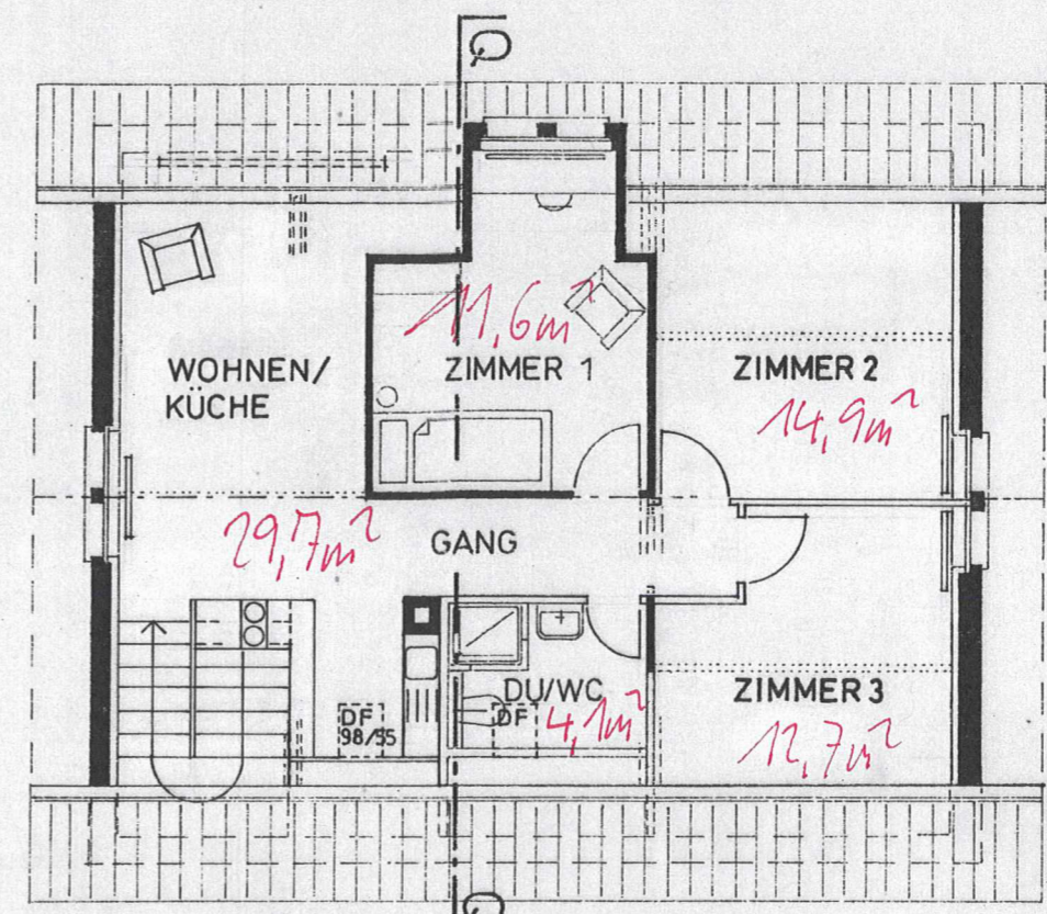
DACHGESCHOSS Total 73,0m 2
