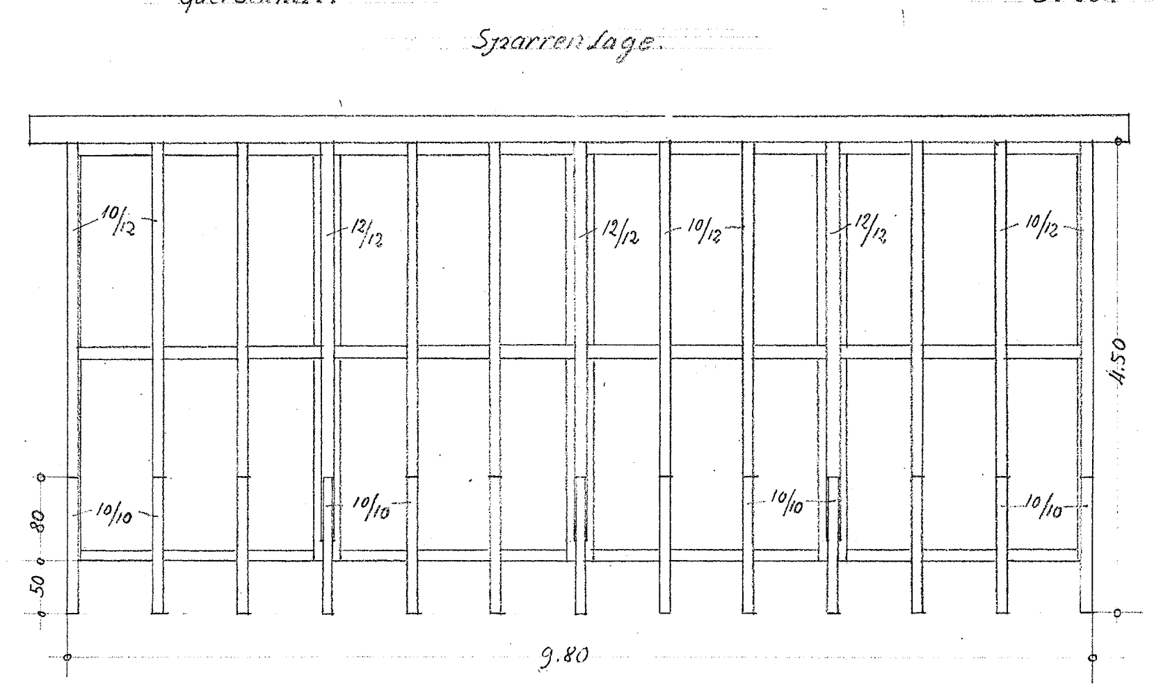
Dachkonstruktion.
