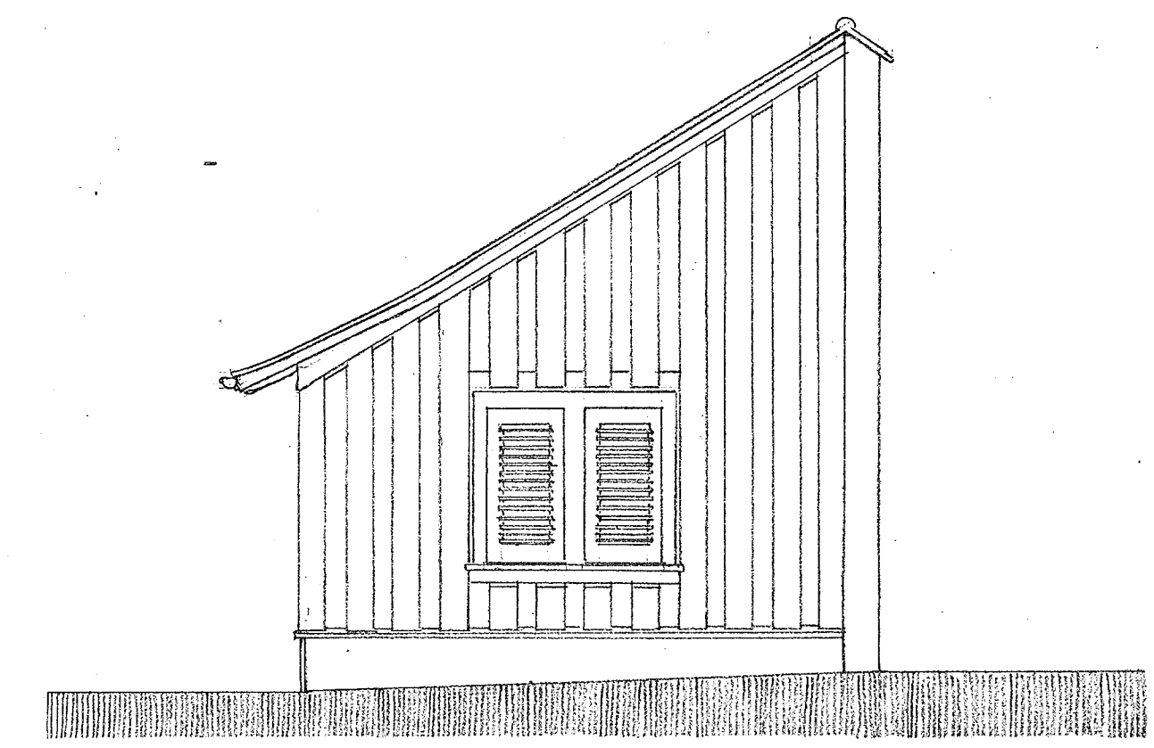
Seiten-Ansicht.
