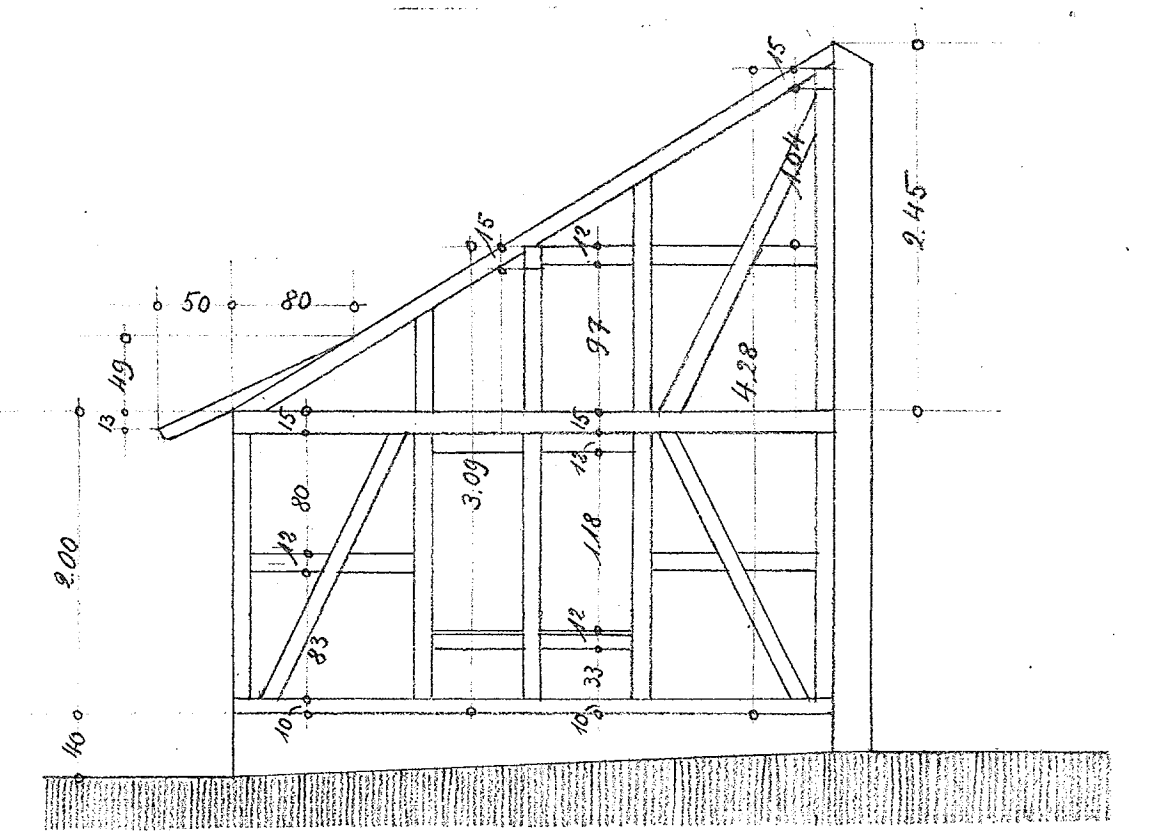
Ansicht der seitl. Fachwerkwände.
