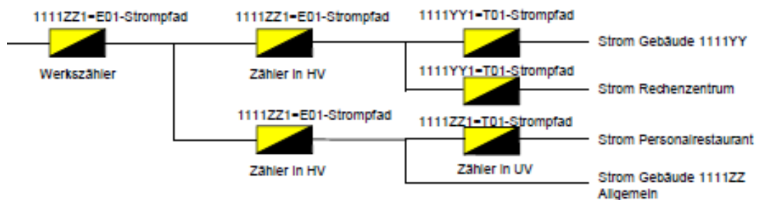
Abbildung 3: Beispiel Darstellung Energiemessschema (Quelle BBL)
