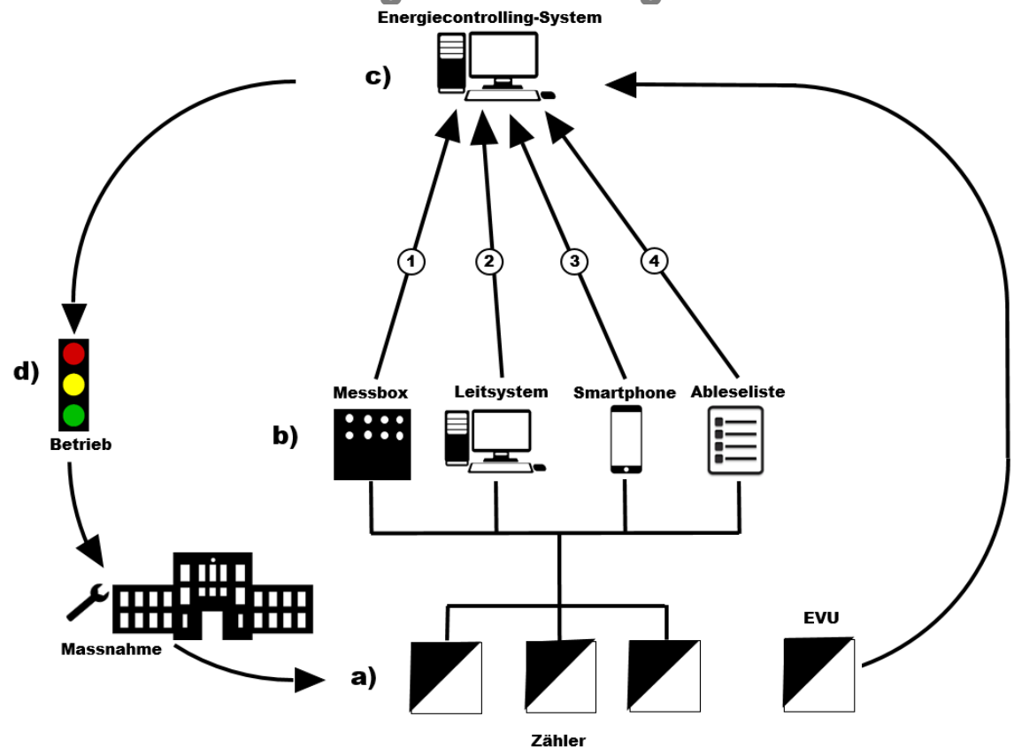
Abbildung 1: Energiecontrolling und Varianten der Energiedatenerfassung
