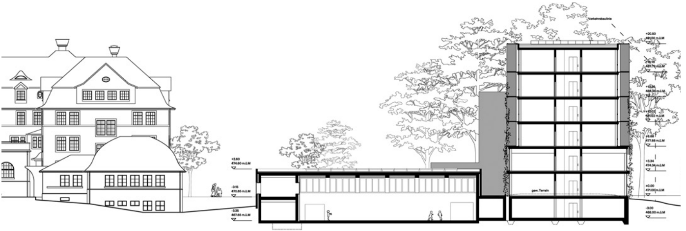
Querschnitt 1:500
