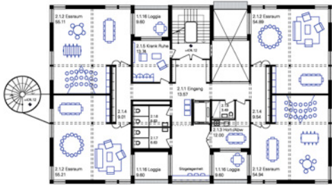
1. Obergeschoss Mittagsgruppen 1:500
