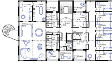
2. bis 4. Obergeschoss Wohngruppen 1:500
