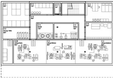
2. Untergeschoss Technik und Facility 1:500
