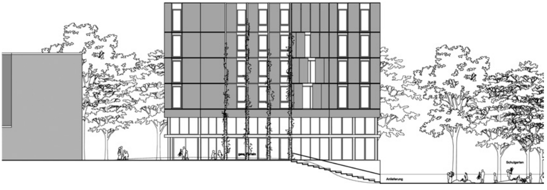
Ansicht Nord 1:500
