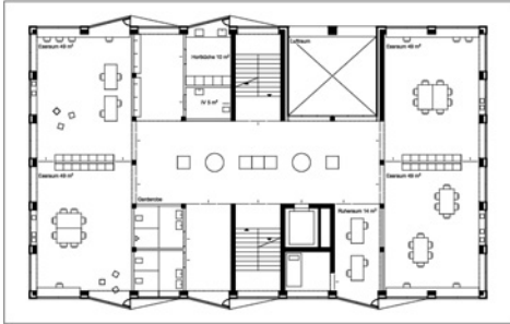
1. Obergeschoss Mittagsgruppen 1:500
