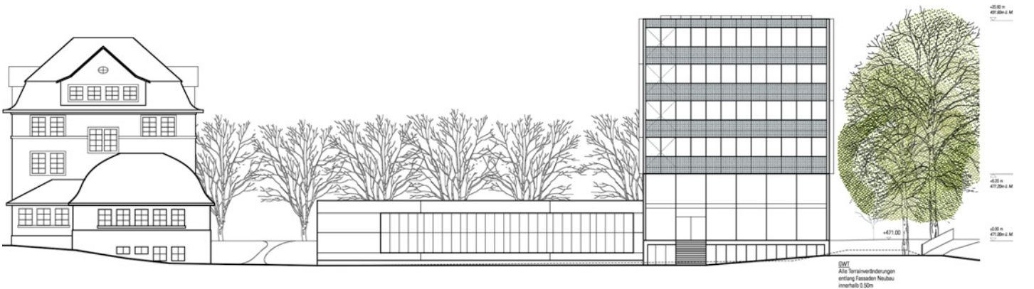
Ansicht West 1:500
