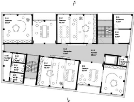
1. Obergeschoss Mittagsgruppen 1:500
