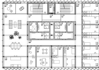
3. bis 6. Obergeschoss Wohngruppen 1:500
