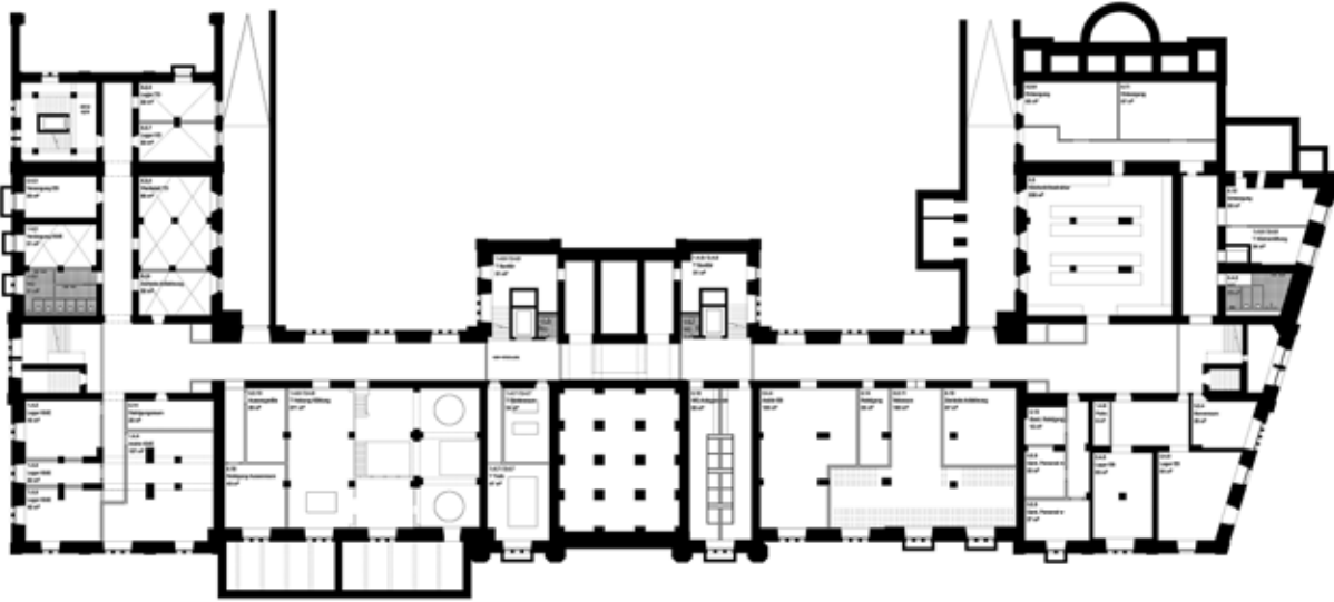
Untergeschoss 1:850
