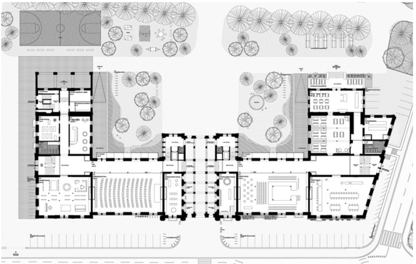
Erdgeschoss 1:850
