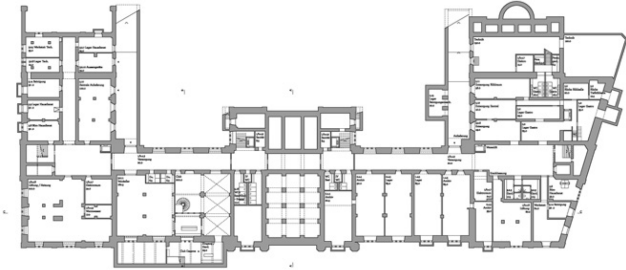
Untergeschoss 1:850
