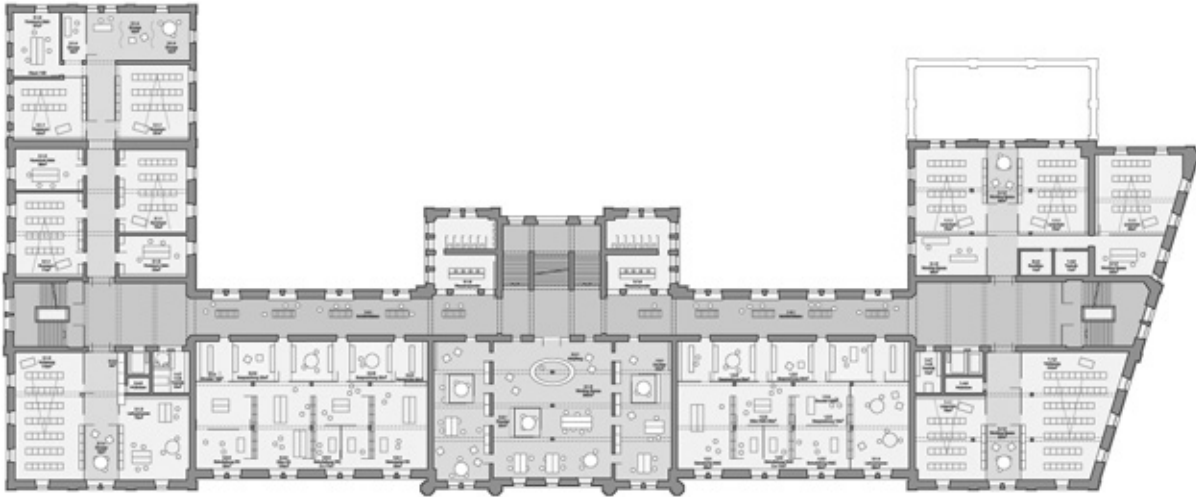
1. Obergeschoss 1:850
