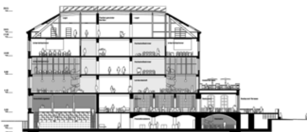
Querschnitt 1:850
