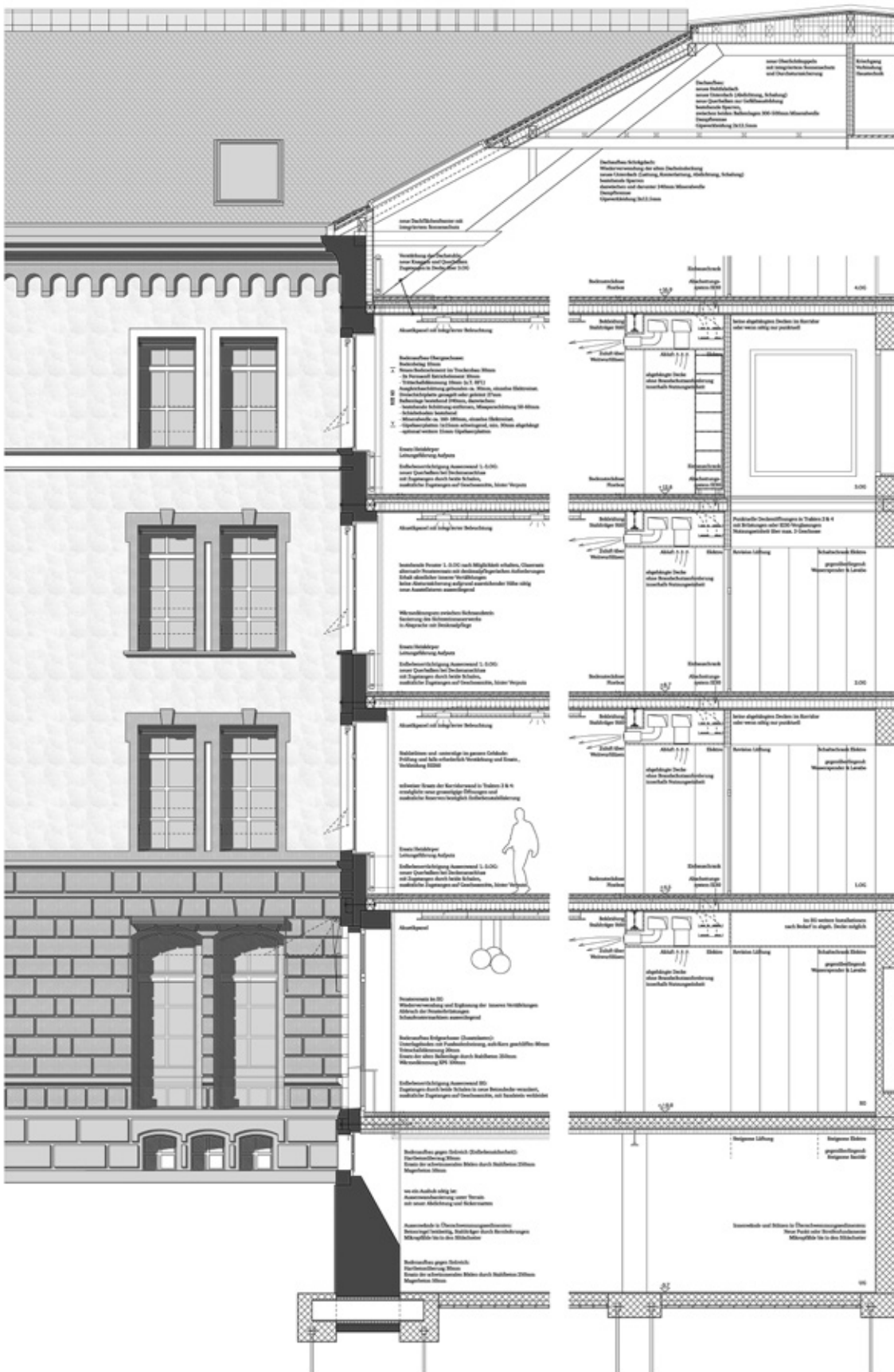
Konstruktionsschnitt mit Teilansicht 1:125
