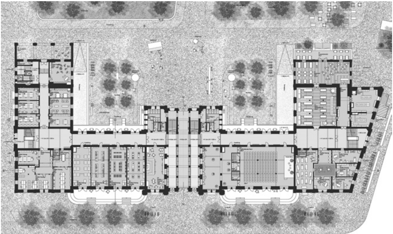
Erdgeschoss 1:850
