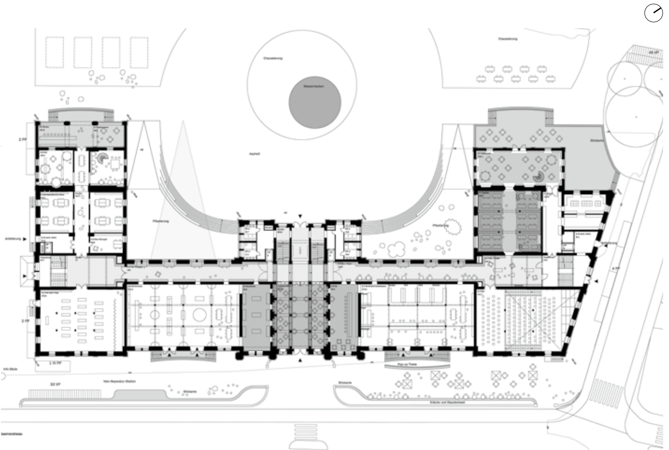
Erdgeschoss 1:850
