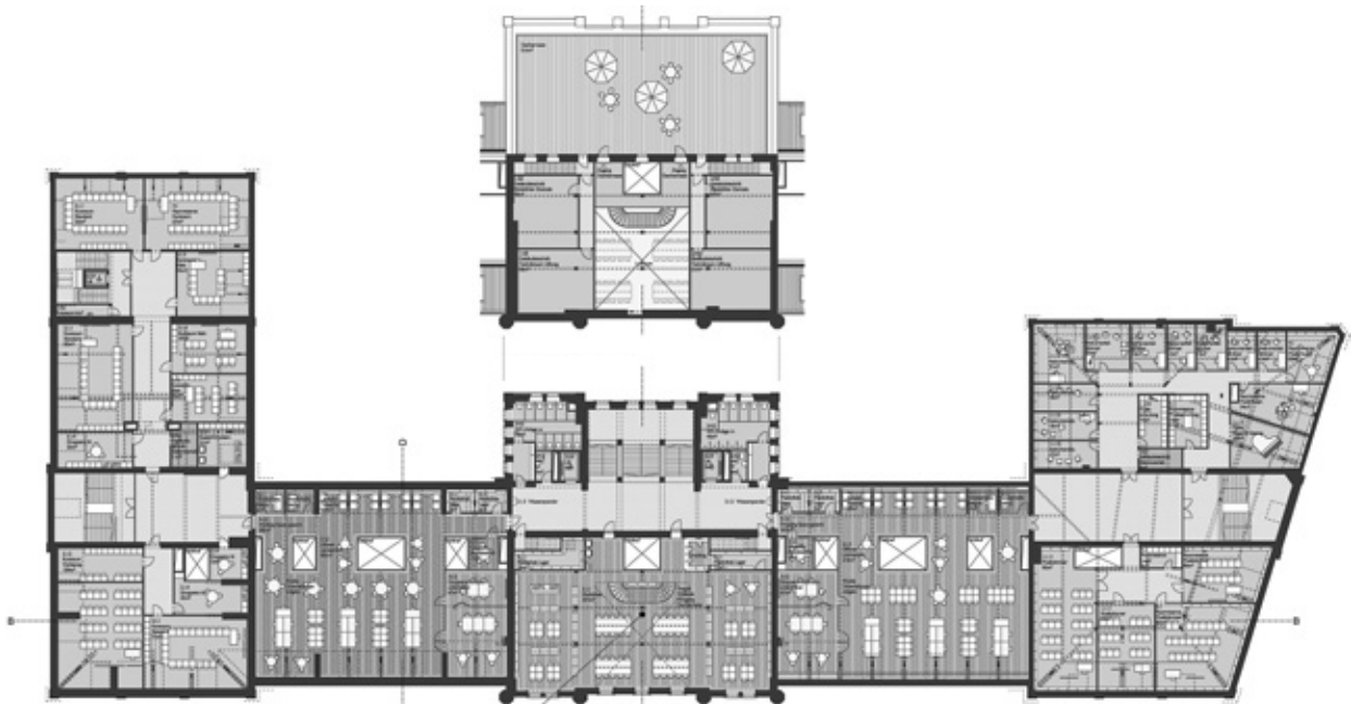
4./5. Obergeschoss 1:850
