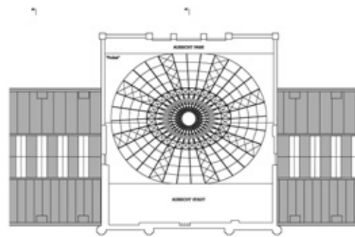
Dachaufsicht 1:850
