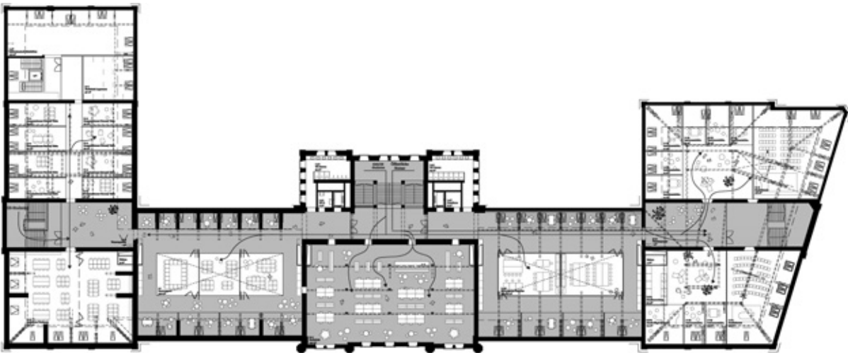
4. Obergeschoss 1:850
