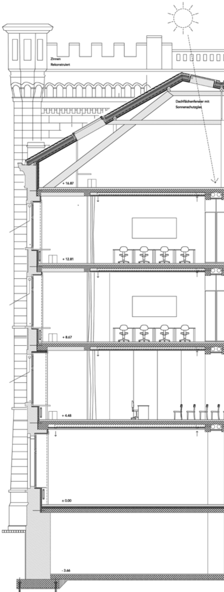
Konstruktionsschnitt 1:125
