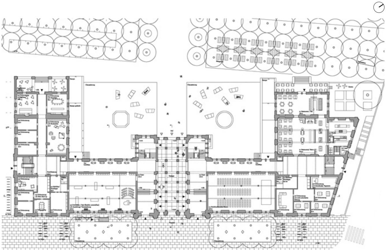
Erdgeschoss 1:850
