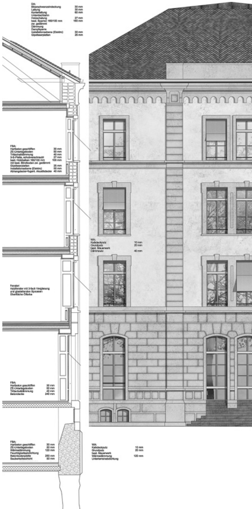
Konstruktionsschnitt mit Teilansicht 1:125
