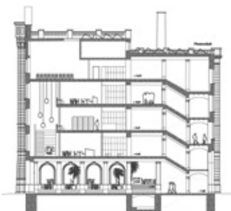
Querschnitt Mittelrisalit 1:850
