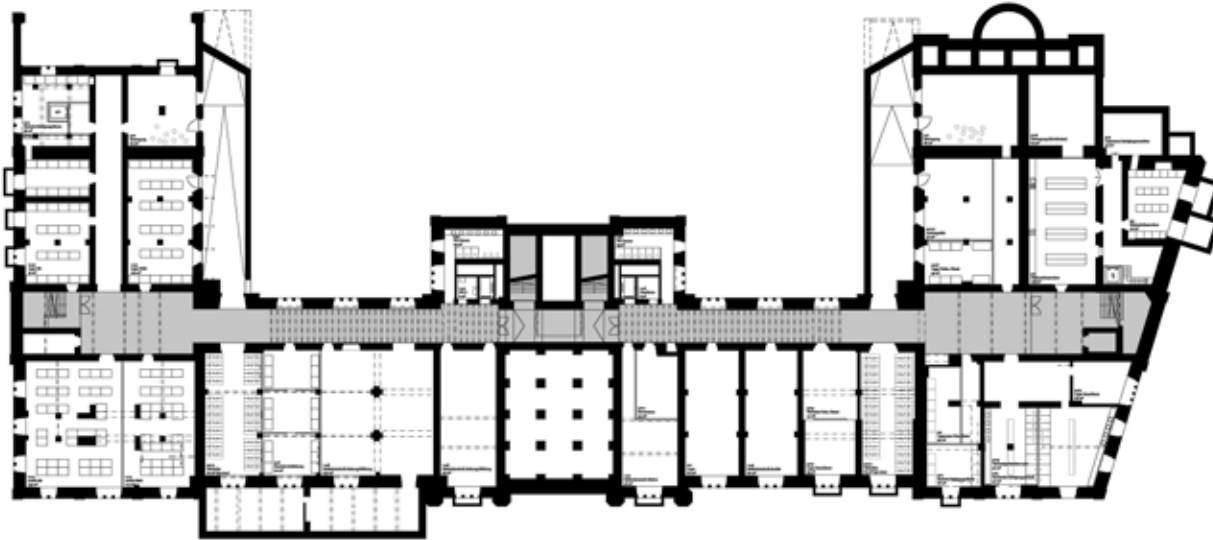
1. Untergeschoss 1:850
