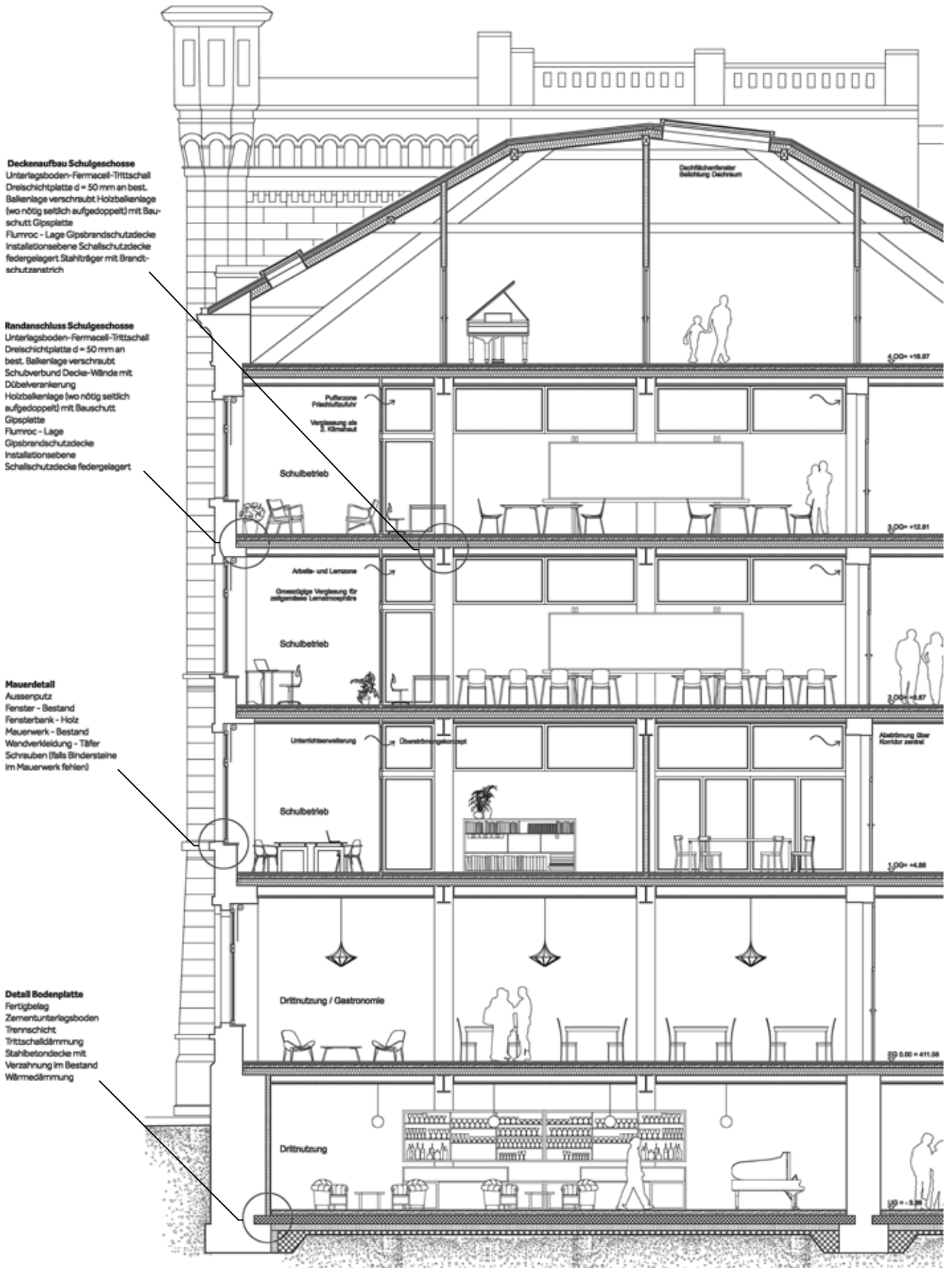
Konstruktionsschnitt 1:125
