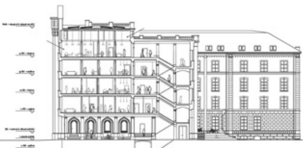
Querschnitt 1:850
