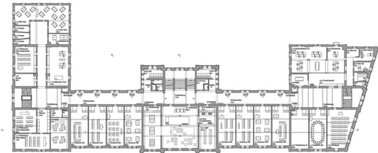
2. Obergeschoss 1:850
