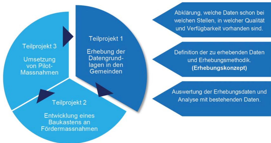
Abbildung 5 Projektstruktur
