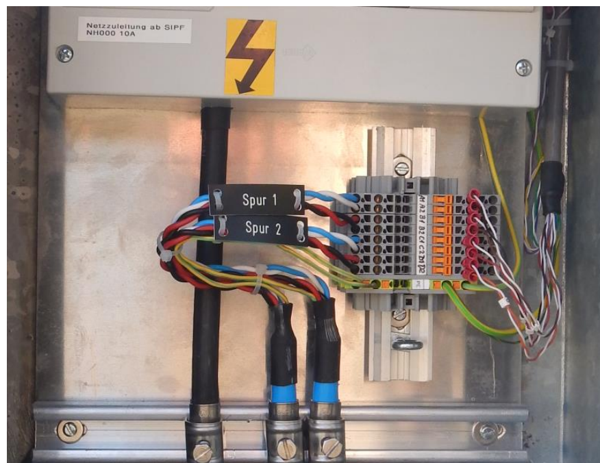
Abbildung 19: Aufschaltung der Schleifenzuleitungskabel auf der Elektrogrundplatte Version 2023 im Messmasten
