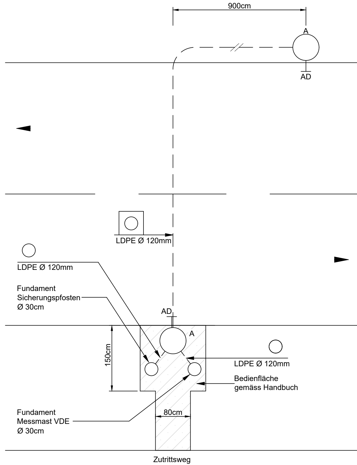
Grundriss 1:50
