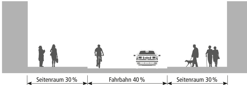
Abb. 6 Als angenehm empfundene Proportionierung des Strassenraums im Verhältnis 3 : 4 : 3 (Eigene Darstellung aufgrund der Richtlinien für die Anlage von Stadtstrassen RASSt 06)
