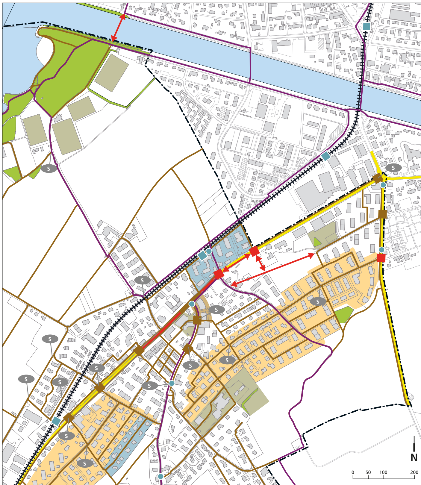
Abb. 12 Darstellungsbeispiel Analyseplan Fusswegnetz (Ausschnitt)
