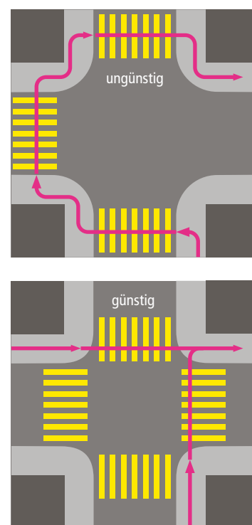
Abb. 32 Querungen über jeden Kreuzungspunkt vermeiden Umwege und Wartezeiten
