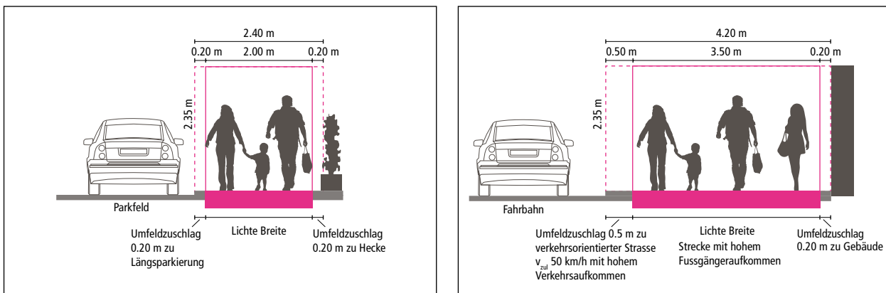
Abb. 8 Resultierende Gesamtbreite aus der Addition von Lichte Breite und Umfeldzuschlag
