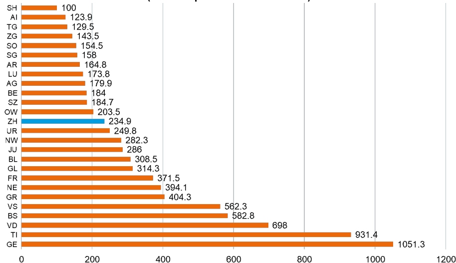
Vergleich Kantone (Inzidenz pro 100'000 Einwohner)
