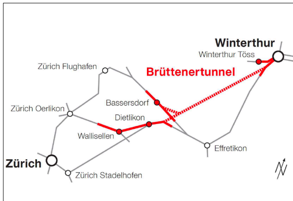
Abb. 4.2b (li.): Übersicht Projekt MehrSpur Zürich – Winterthur mit Kernstück Brüttenertunnel, SBB (2020)
