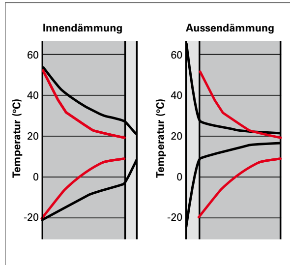
Temperaturverhältnisse in der Konstruktion: ungedämmt (rot), mit Innen- und mit Aussendämmung (Abb. 26)
